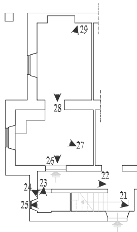
PLANIMETRIA FABBRICATO
