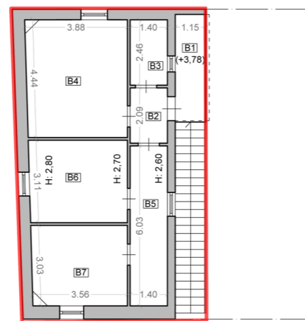
PIANTA PIANO PRIMO - C.F. F25 P731 S2 scala 1:200
