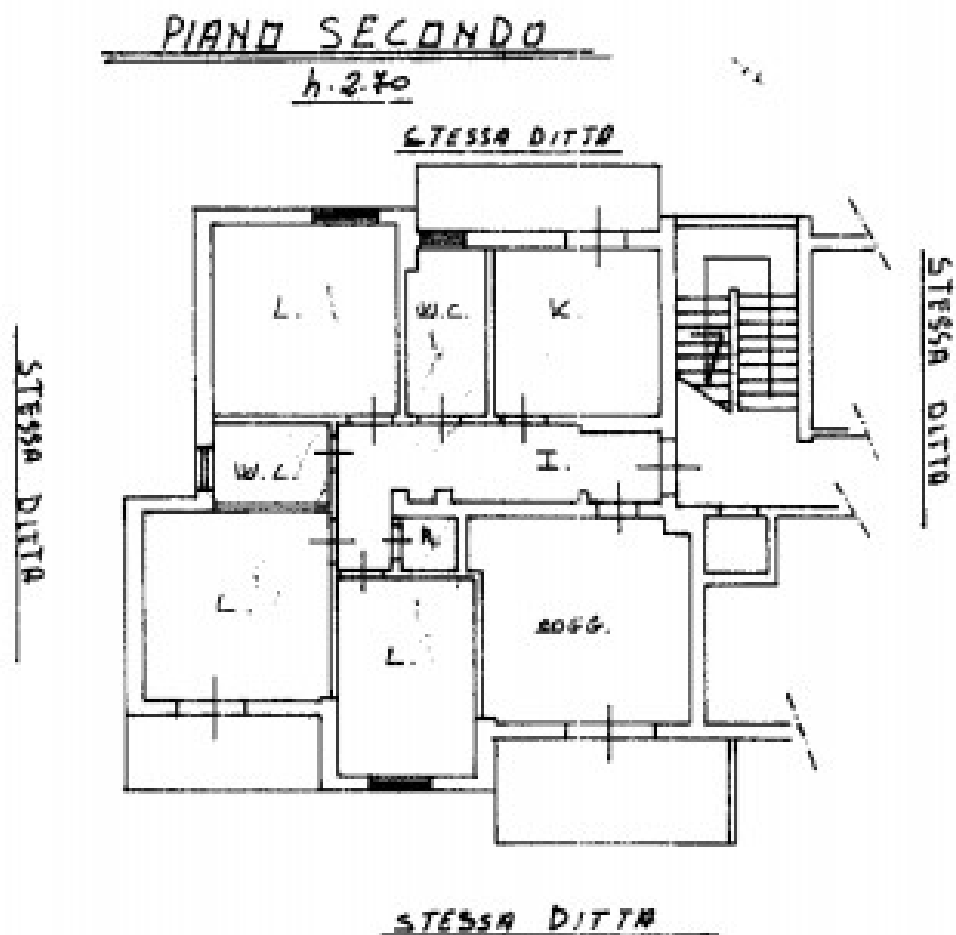
Figura 4: estratto planimetrico immobile
