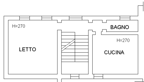
PIANO PRIMO
