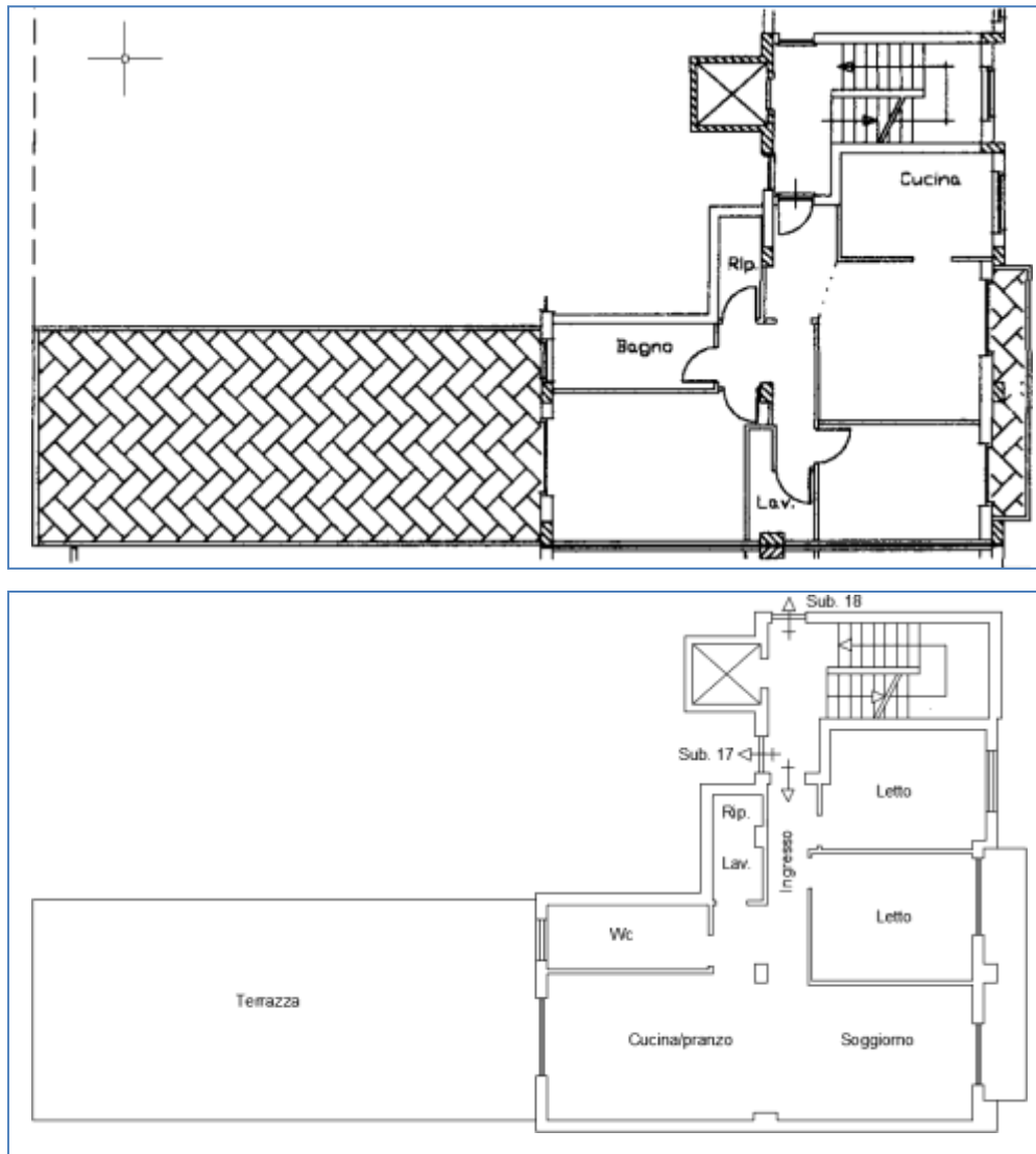
Figure 8 – Confronto tra la Planimetria catastale (in alto) e restituzione grafica dello stato dei luoghi (in basso)
