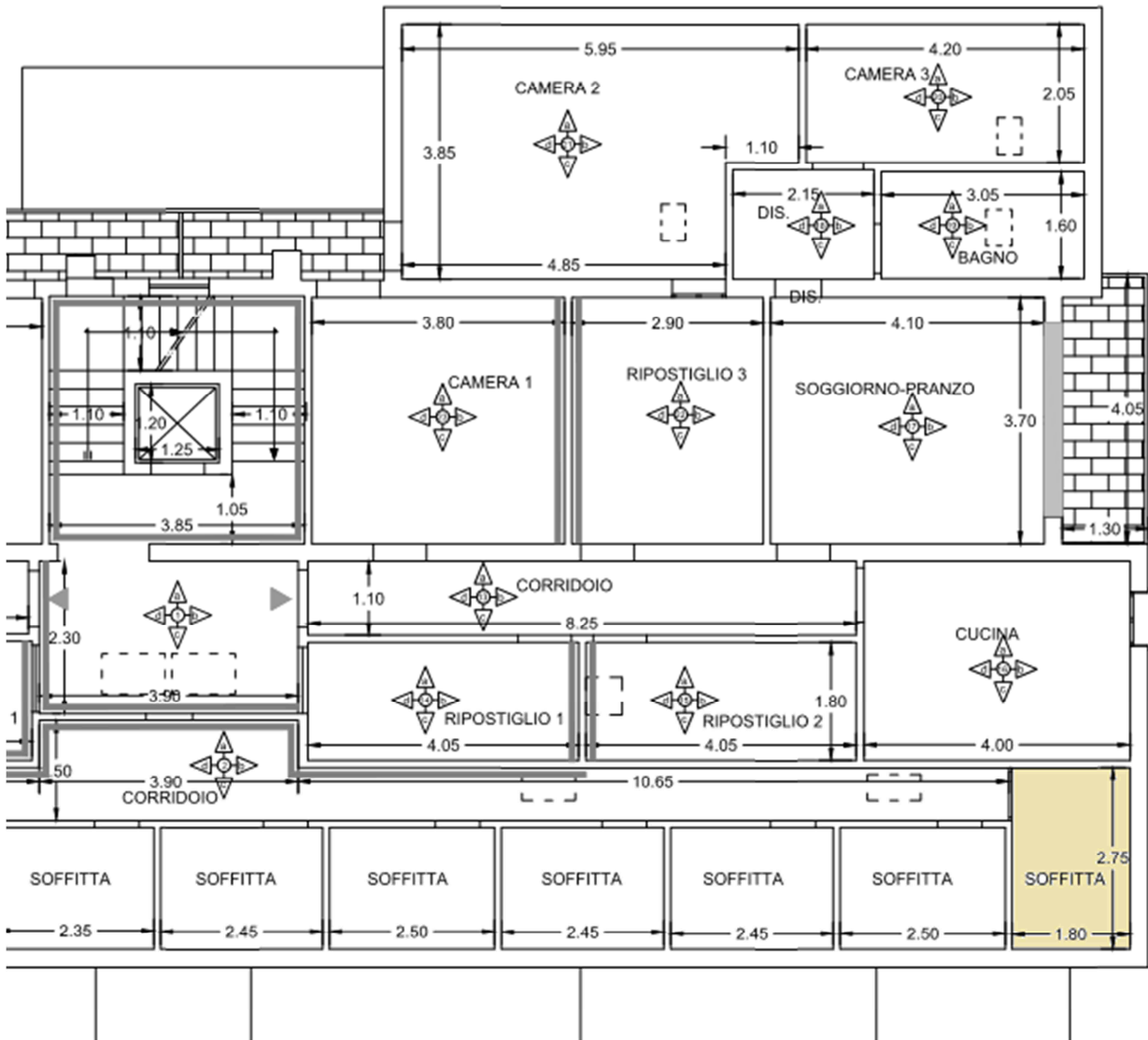
SOFFITTA PIANO SOTTOTETTO STATO DI PROGETTO SCIA Pratica edilizia N. 77/2014
