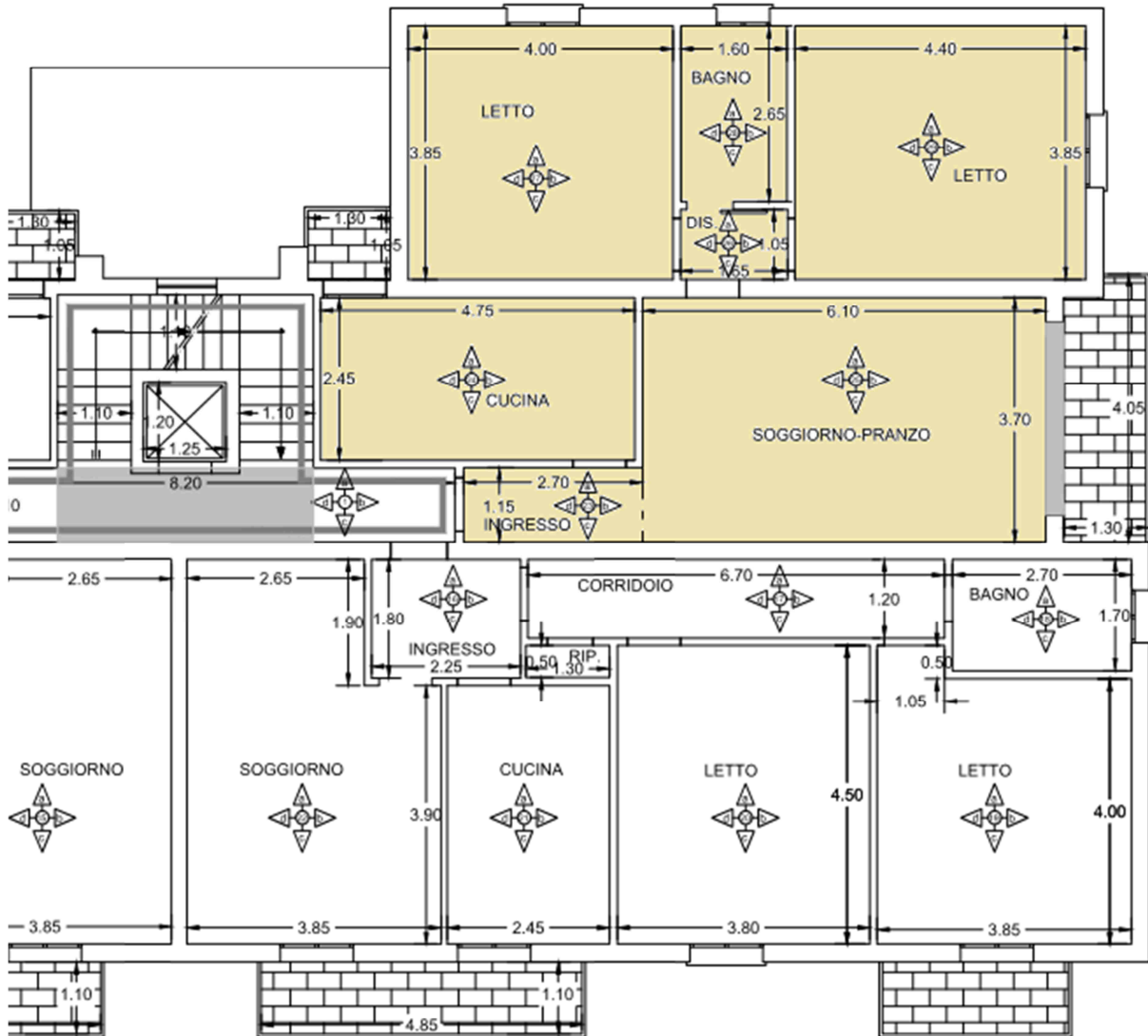
APPARTAMENTO PIANO TERZO STATO DI PROGETTO SCIA Pratica edilizia N. 77/2014
