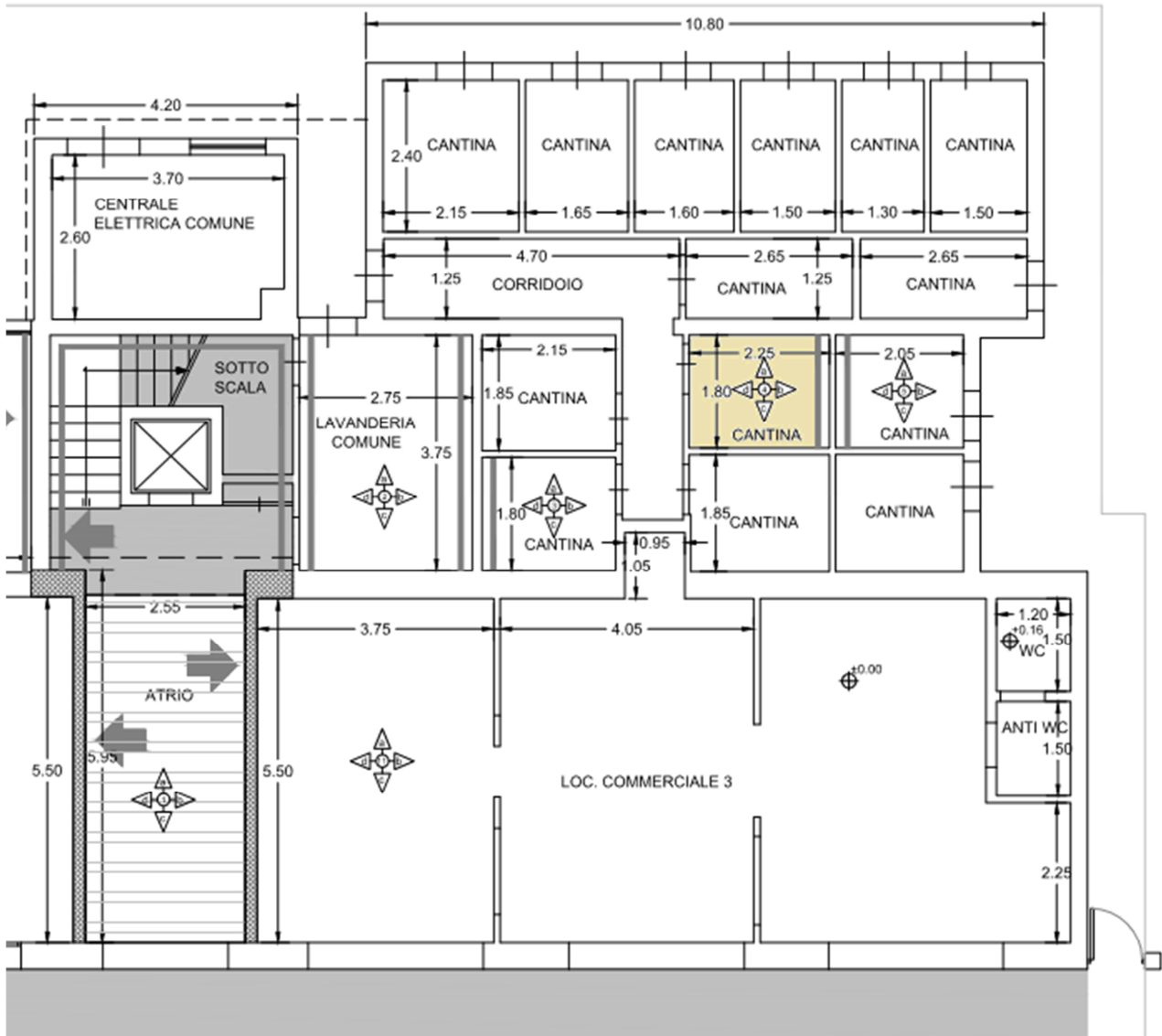
CANTINA PIANO TERRA STATO DI PROGETTO SCIA Pratica edilizia N. 77/2014
