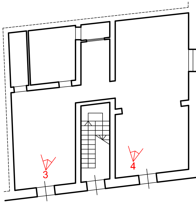
Piano Terra Stato di Fatto
