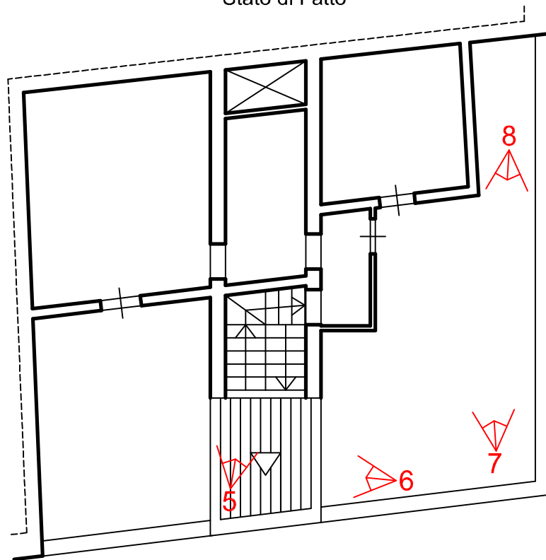
Piano Quarto Stato di Fatto
