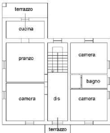
PIANO PRIMO H=2.90
