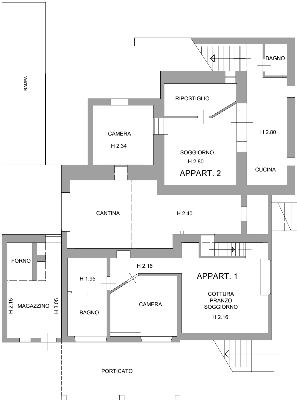
PIANTA PIANO TERRA/SEMINTERRATO Scala 1.100
