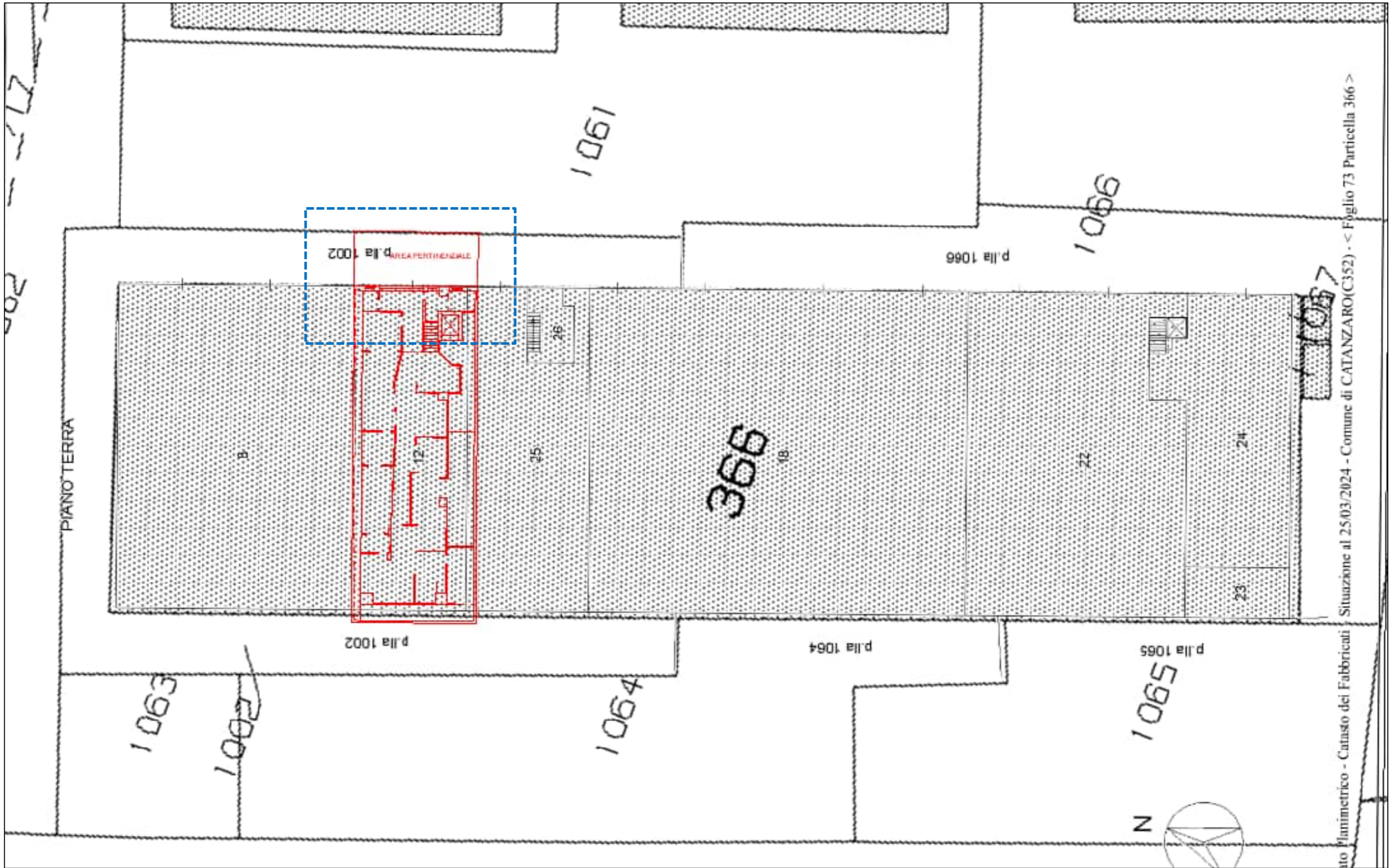
Figura 12 - Sovrapposizione tra la planimetria da rilievo del subalterno 12, elaborato planimetrico della particella 366 ed estratto di mappa catastale del foglio 73 – Individuazione area pertinenziale del subalterno 12
