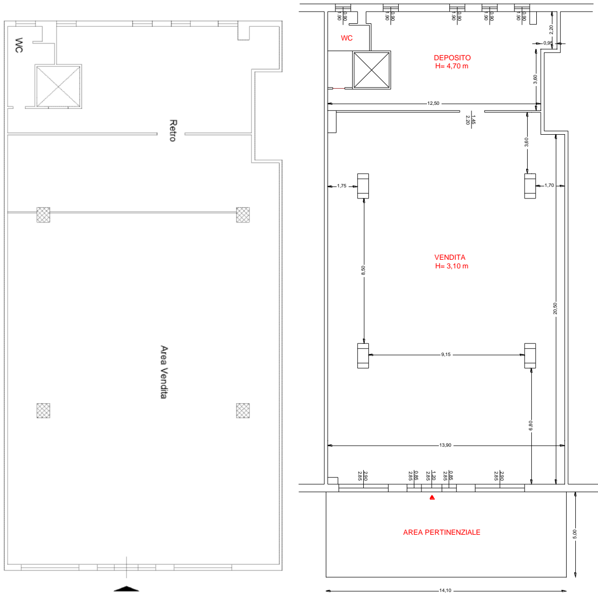
Figura 26 - Raffronto planimetria catastale (a sinistra) e da rilievo (a destra) - Subalterno 27
