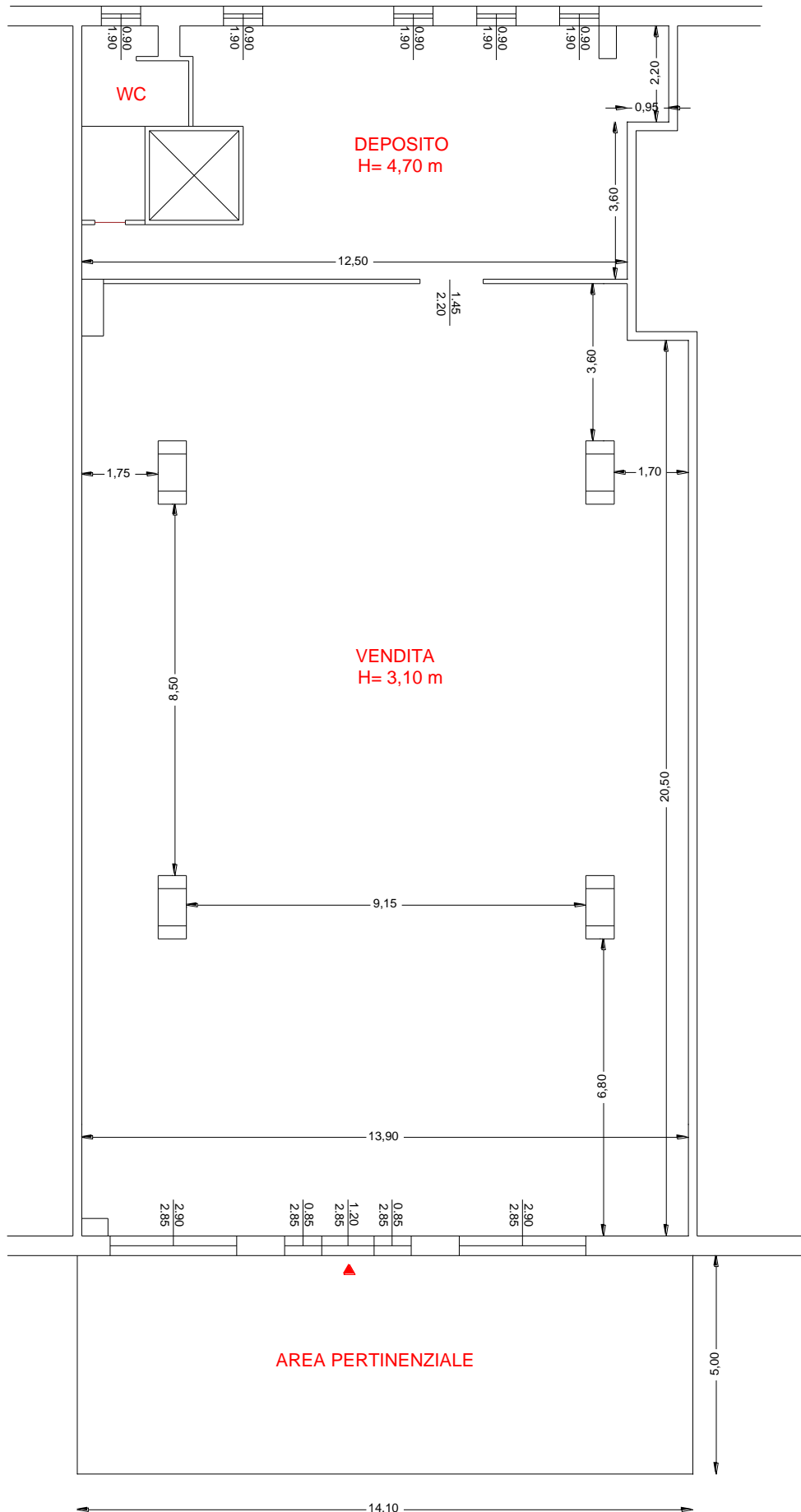
Figura 21 - Planimetria da rilievo subalterno 27
