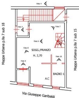
PIANTA PIANO PRIMO (H.2,70)
