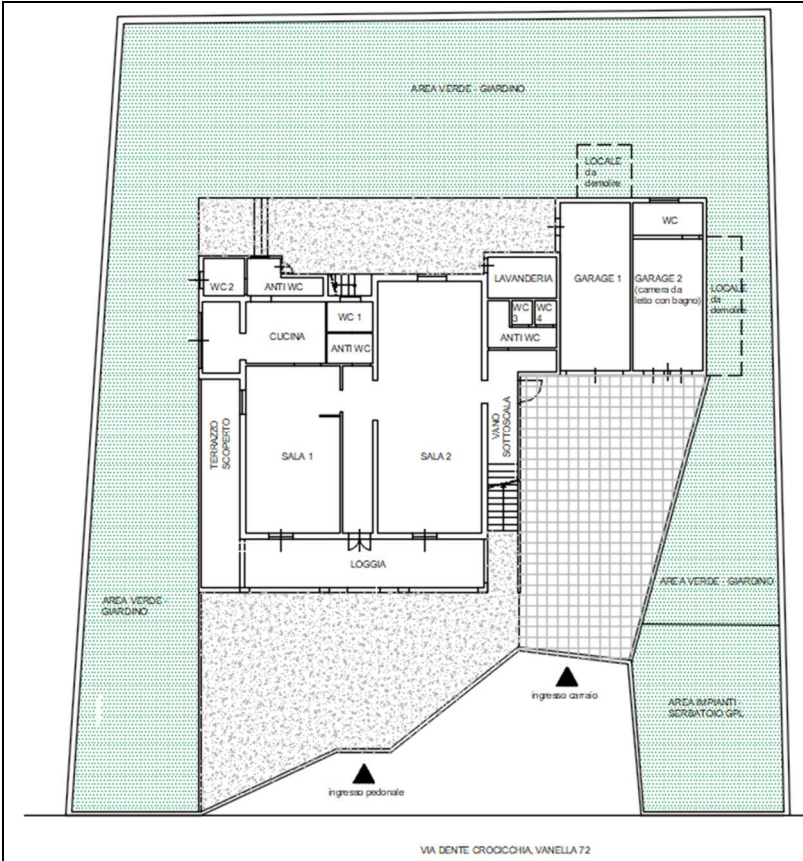
Planimetria piano terra (Locale pubblico esercizio – garage 1 – garage 2)
