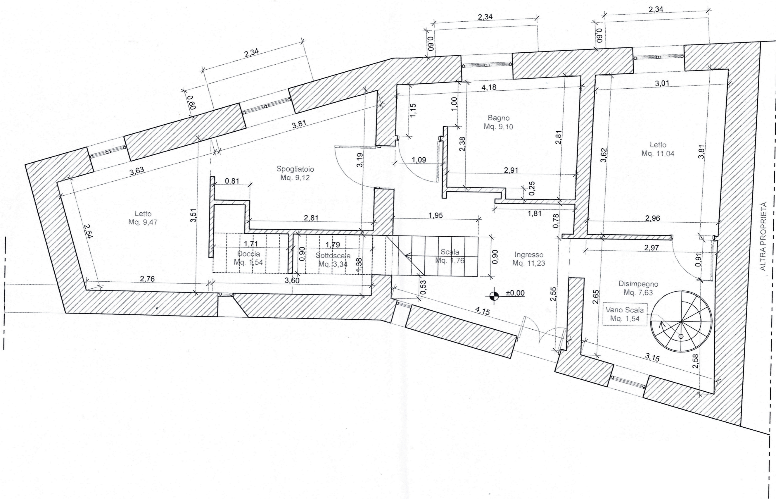
BENE N° 1: PIANTA PIANO TERRA STATO ATTUALE
