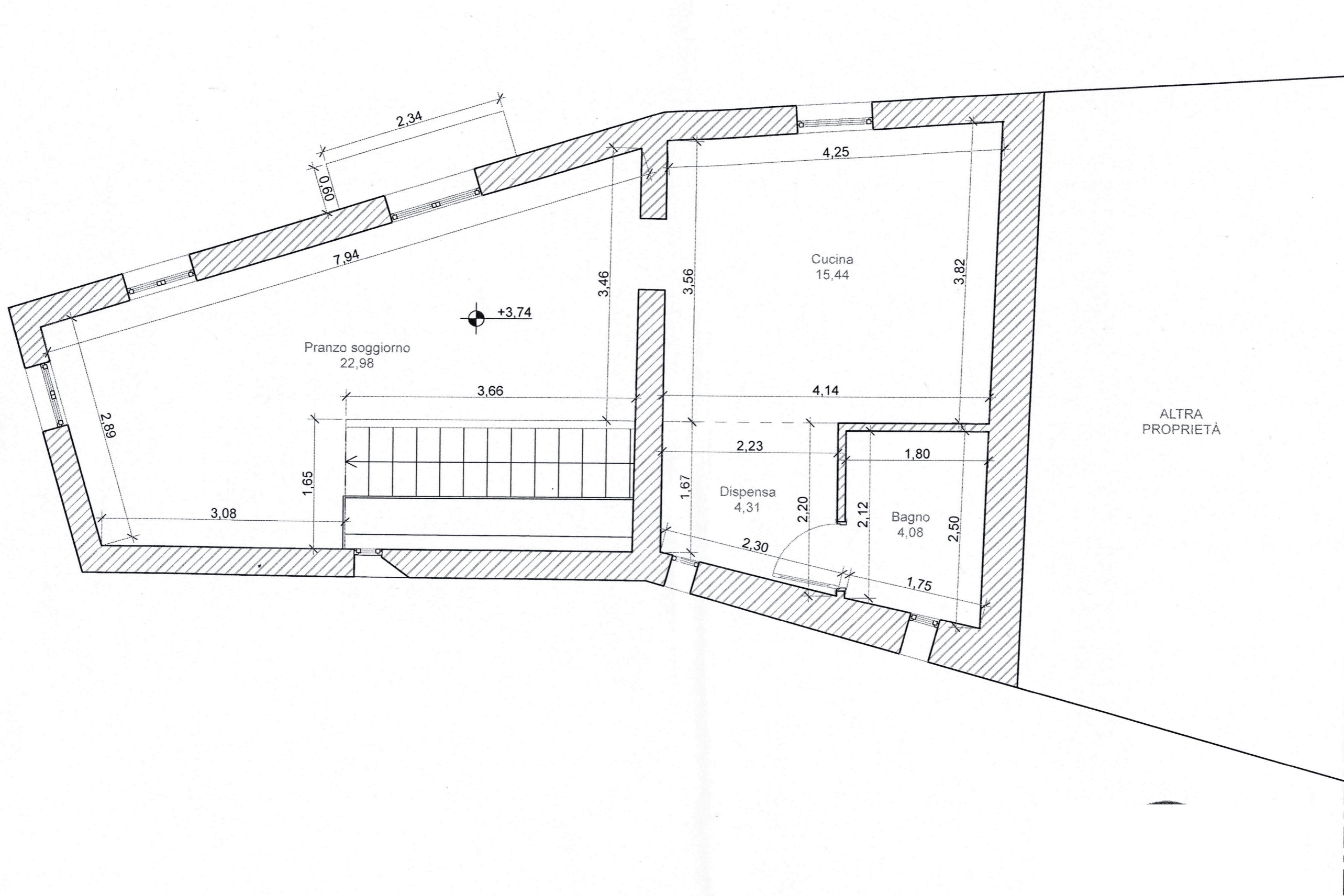
BENE N° 1: PIANTA PIANO TERRA _STATO ATTUALE
