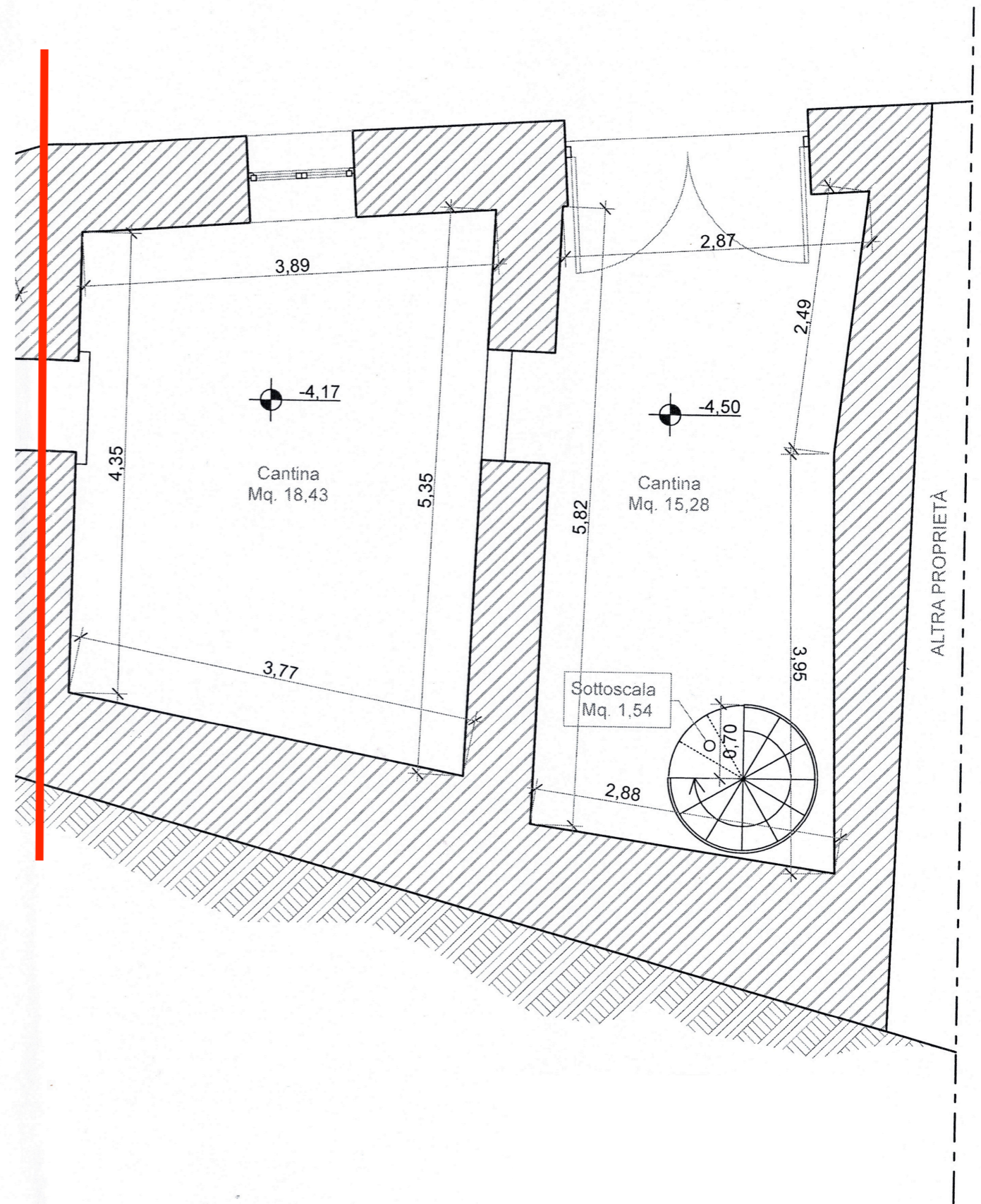
BENE N°1: PIANTA SEMINTERRATO_STATO ATTUALE
