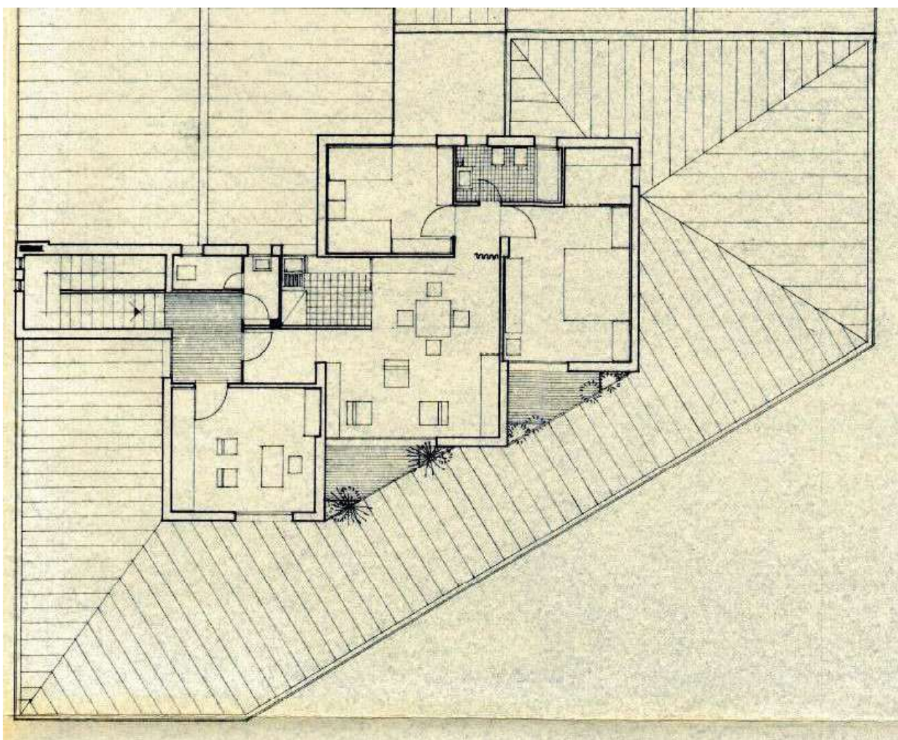
Fig. 2.13 – Pianta Piano Primo Stato Autorizzato (fuori scala)
