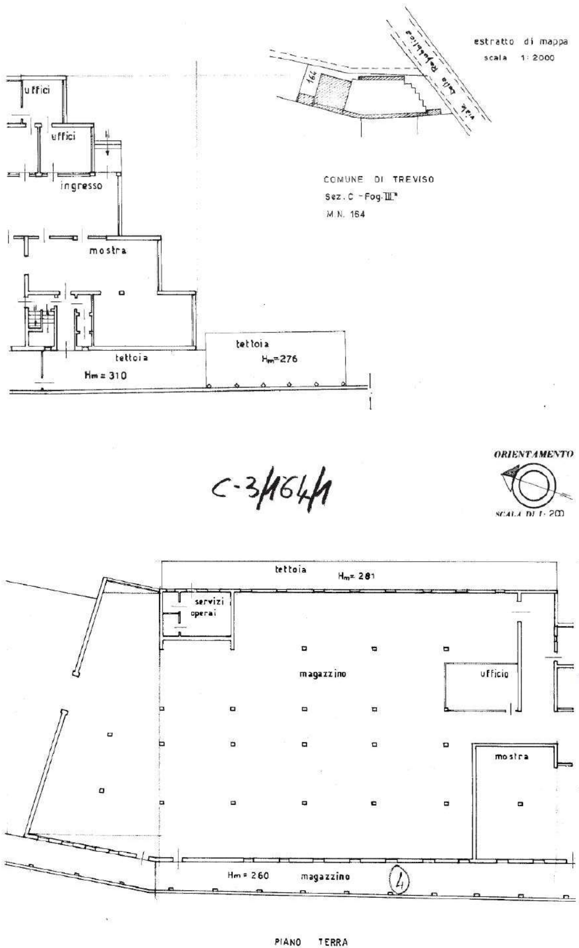
Fig. 2.10 – planim. catastale (fuori scala), sez. C fg. 3 di Treviso, mappale 164 sub 1
