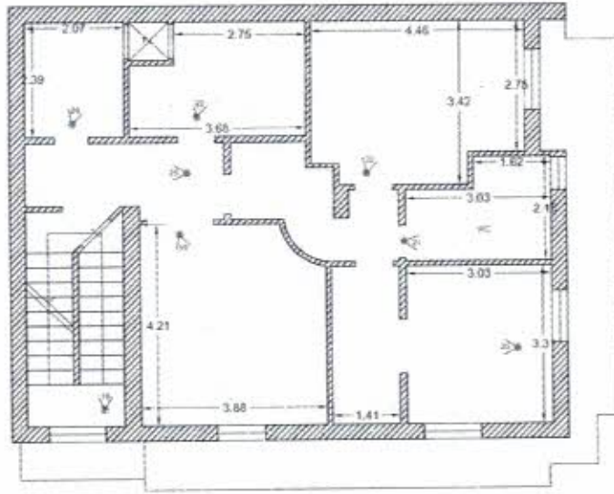
MAPPA PIANO SECONDO
