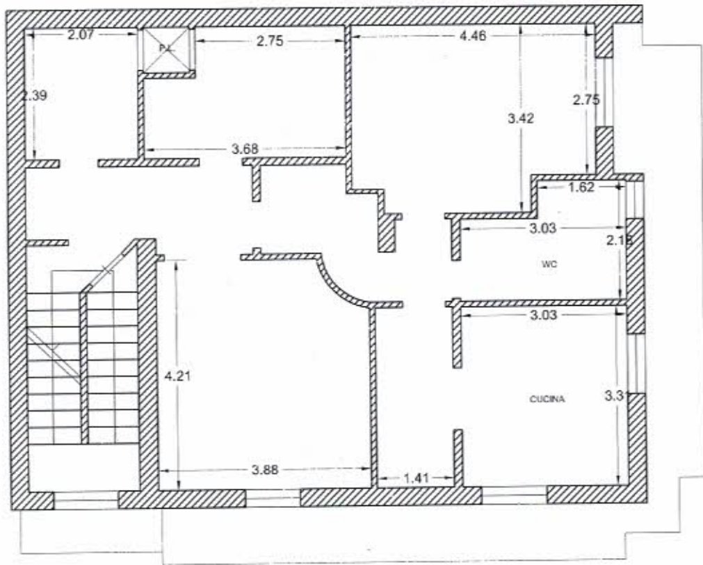
piano piano secondo _ scala 1:100
