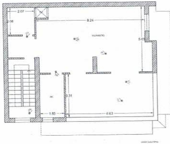
MAPPA PIANO TERZO
