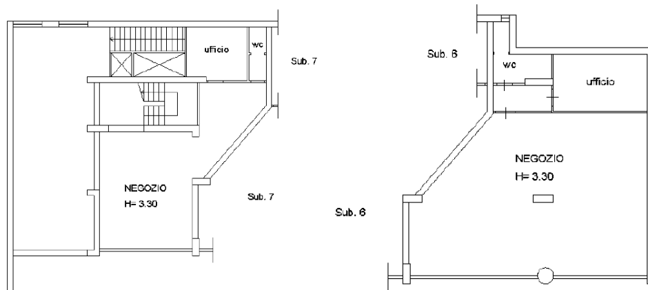
Planimetria catastale Foglio 4 p.lla 5033 sub 6 e sub 7 - piano T
