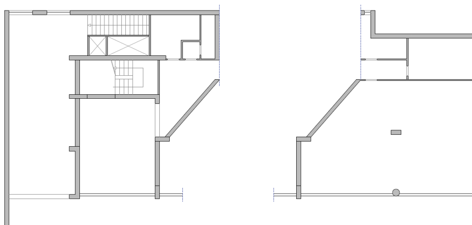
Planimetria dello stato di fatto - piano T
