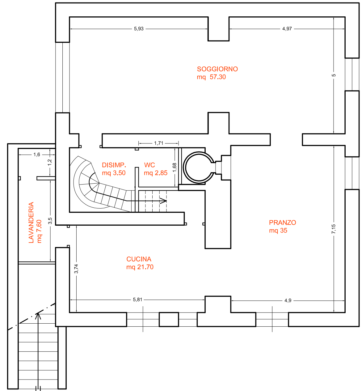
ABITAZIONE Piano Terra
