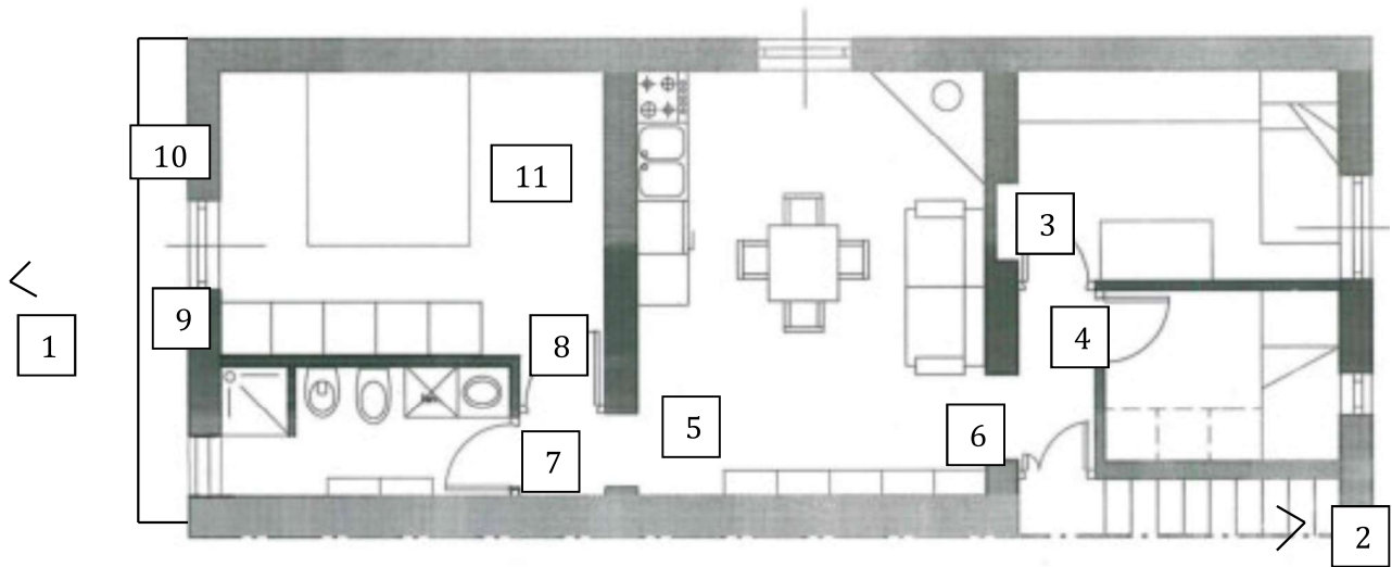
Planimetria Pianta Piano Primo
