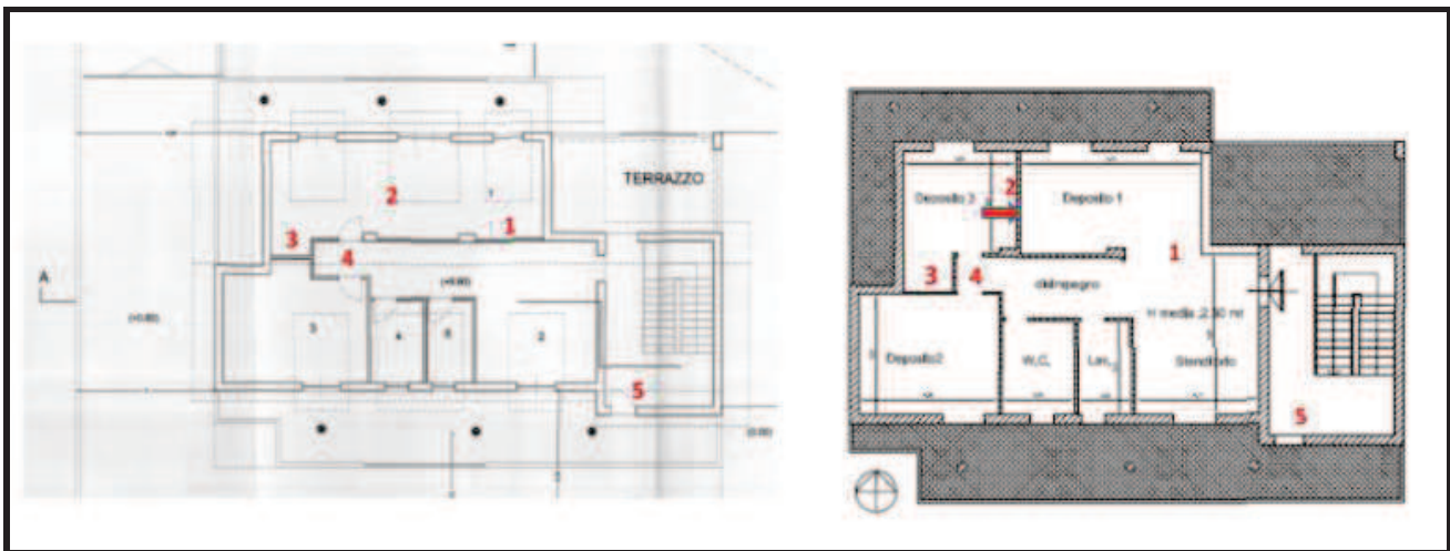
Pianta allegata al P.d.C. n°6 del 2/04/2021
