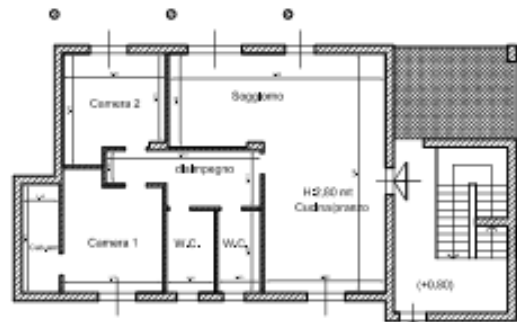
Pianta Piano Terra (+0.80) rapp. 1:100
