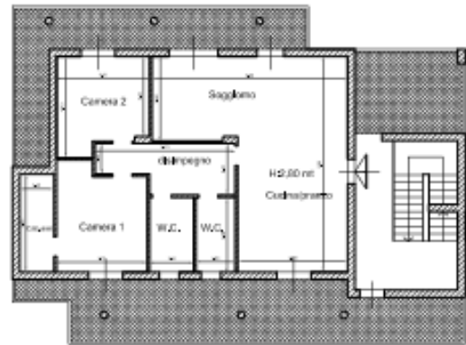
Pianta Piano Primo rapp. 1:100
