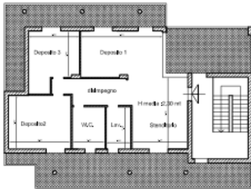
Pianta sottoterra rapp. 1:100
