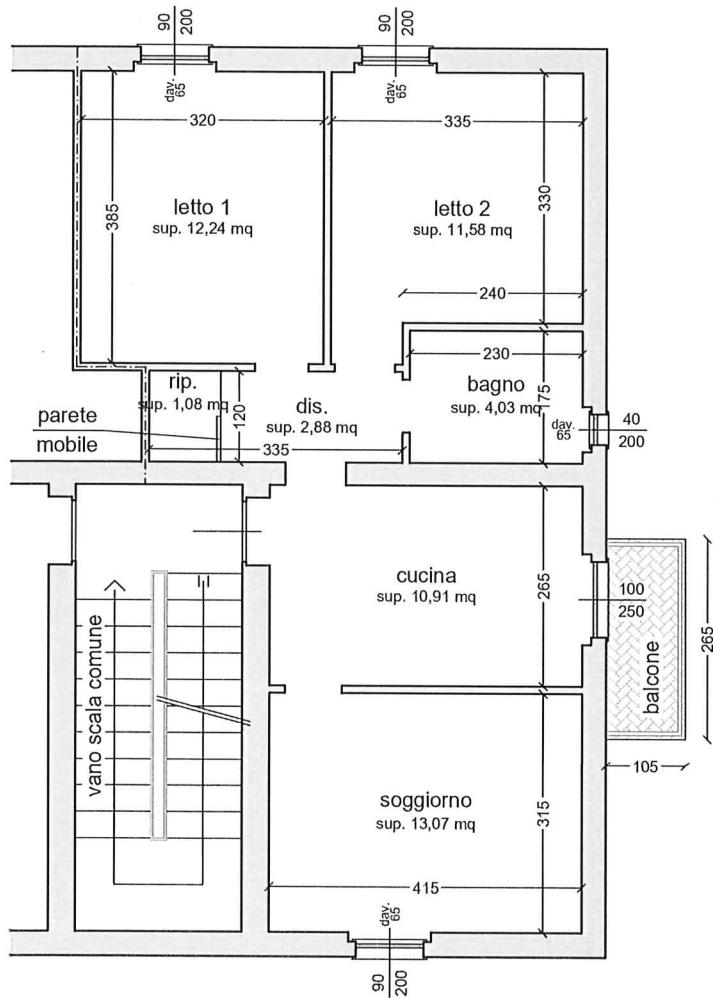
PIANO PRIMO h. 3,05 mt.
