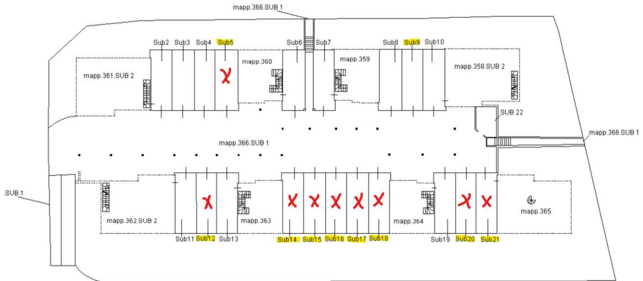
Schema Generale – 358 (semi-interrato)
