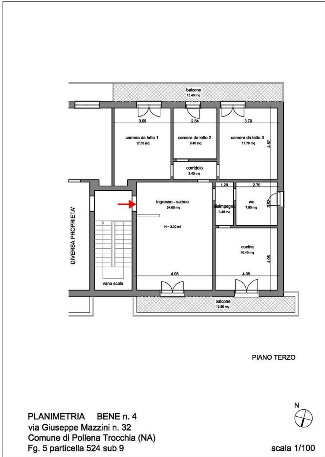
Bene 4 - piano terzo
