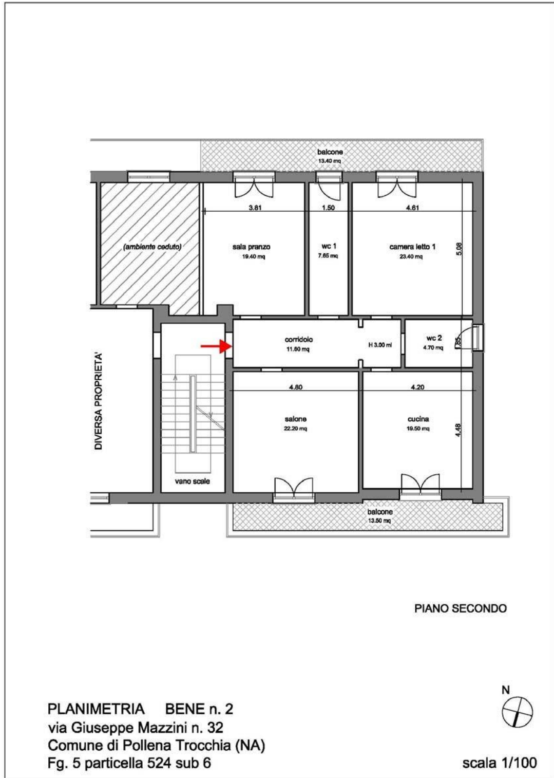
Bene 2 - piano secondo
