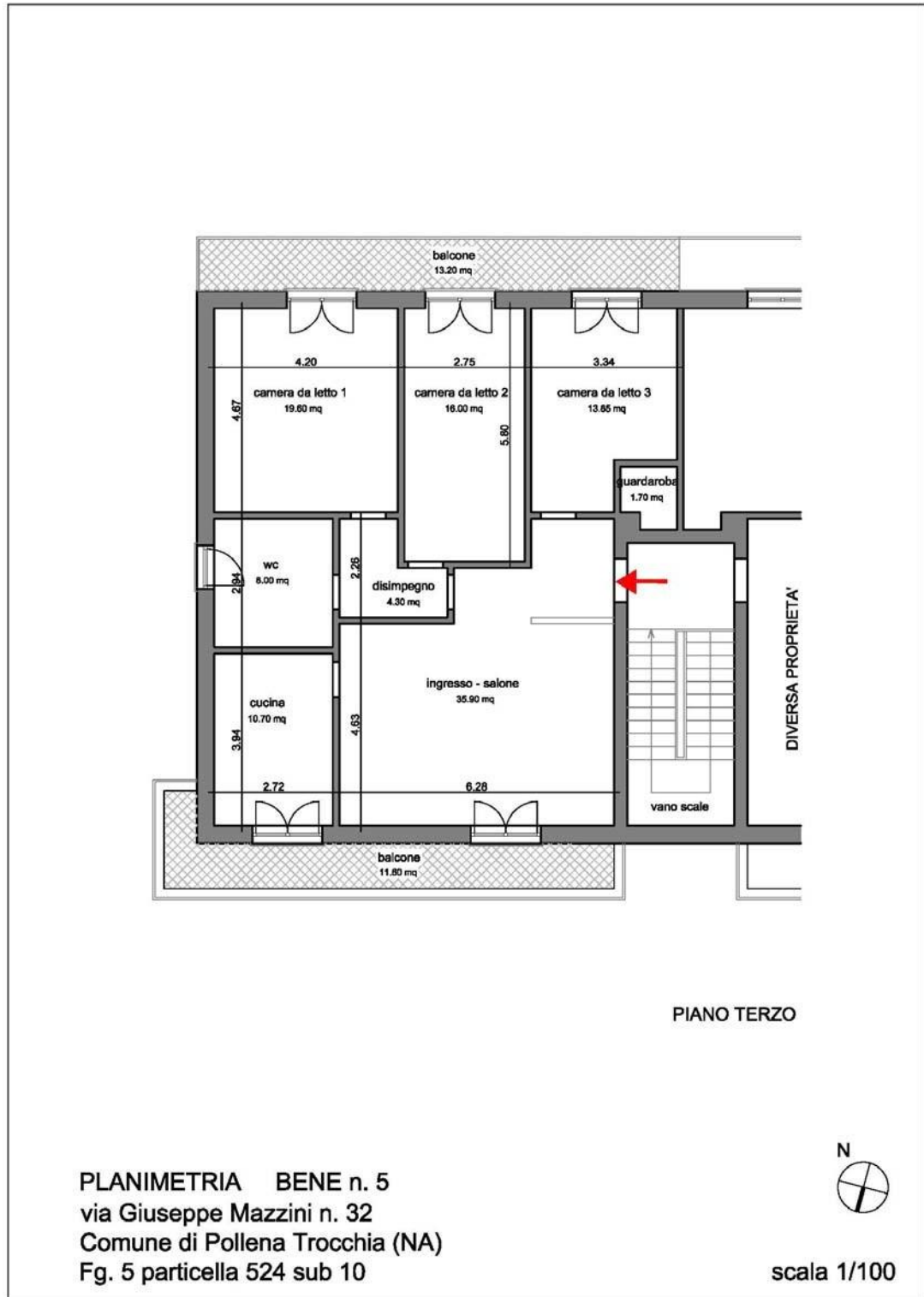
Bene 5 - piano terzo
