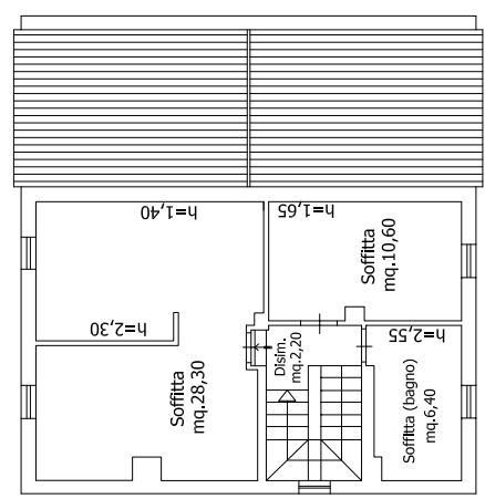
Piano Secondo
