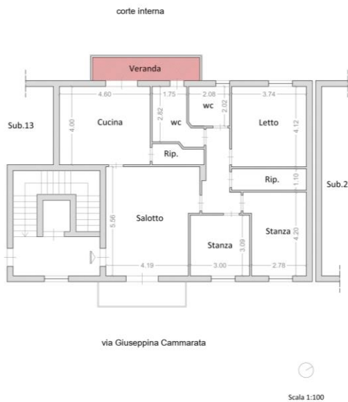
Rilievo dello stato di fatto attuale dell'appartamento con difformità rispetto alla planimetria catastale e al progetto autorizzato (ALL. 8)
