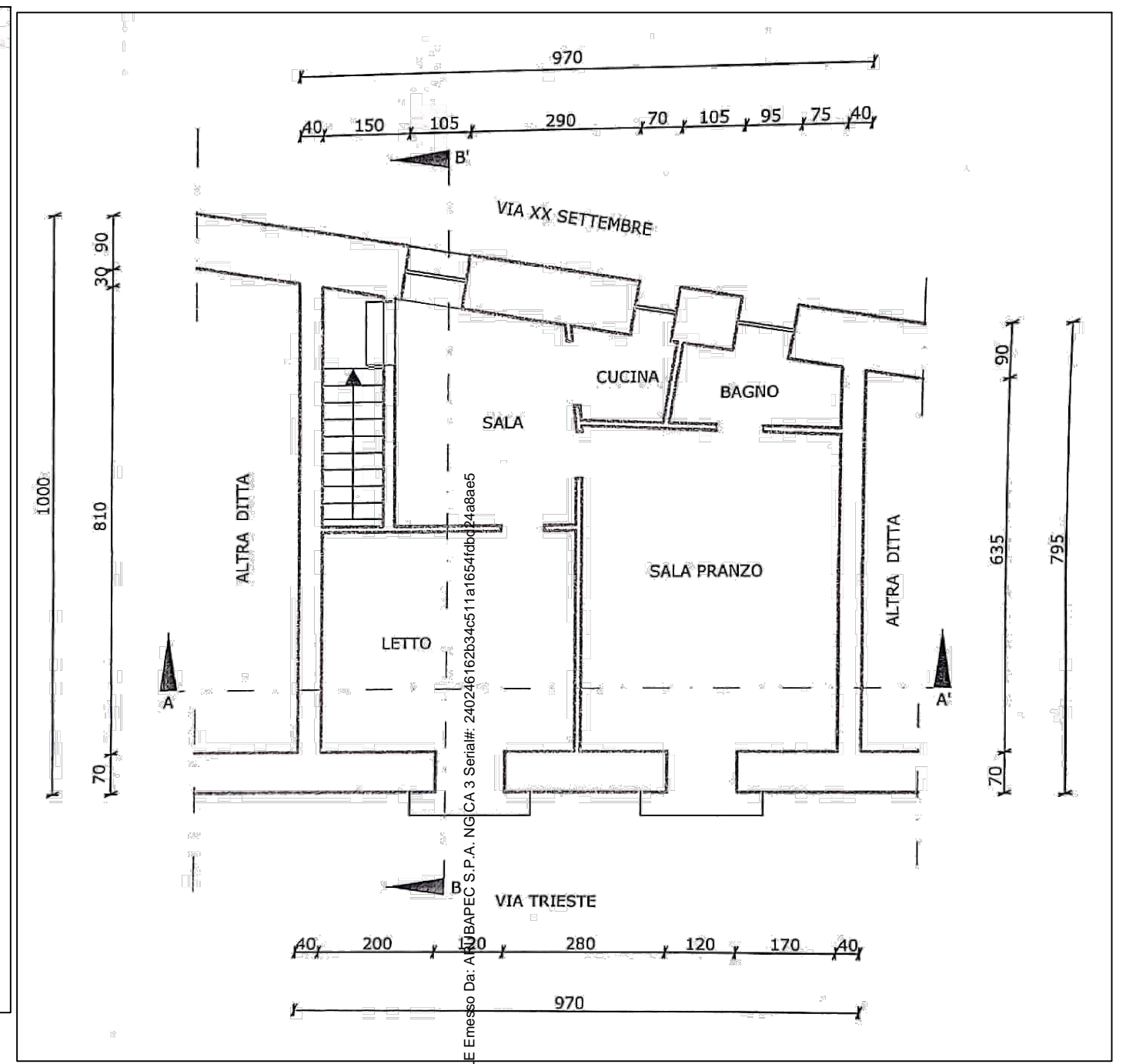
PIANO PRIMO H=3,15m.
