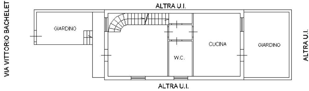
PIANTA PIANO TERRA H= 2,80 MT.
