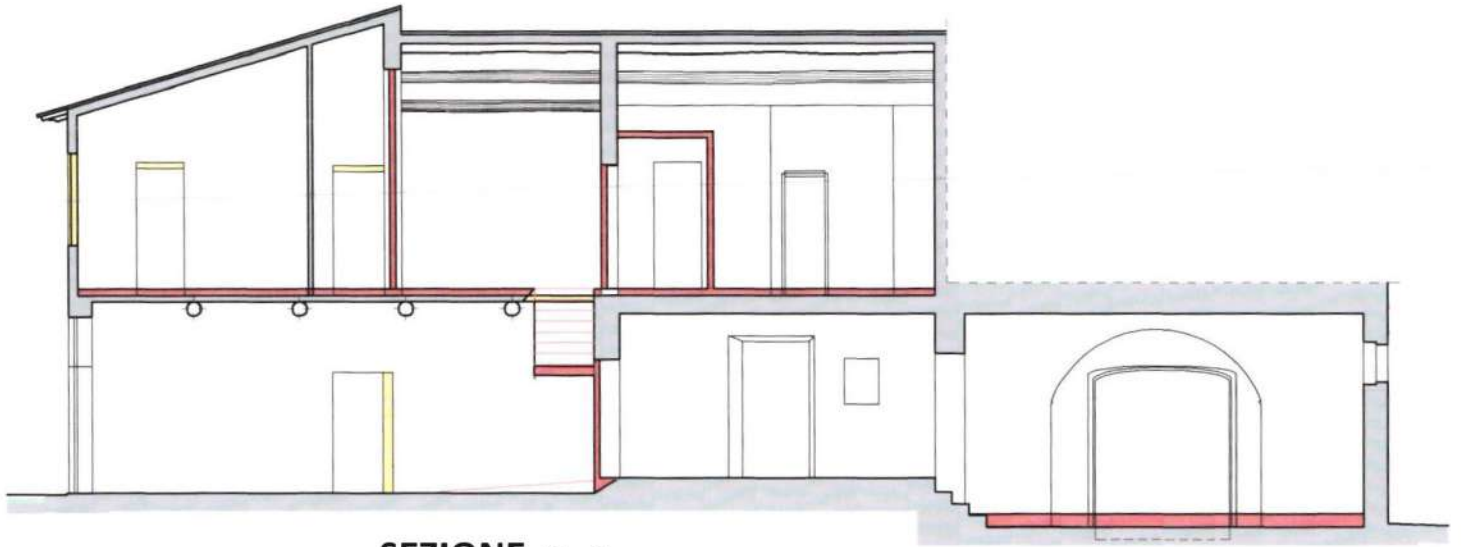
SEZIONE c - c
