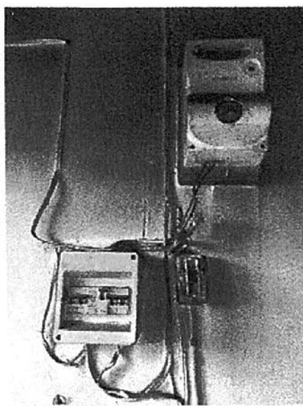
Foto 28 - Particolare dell'impianto elettrico
