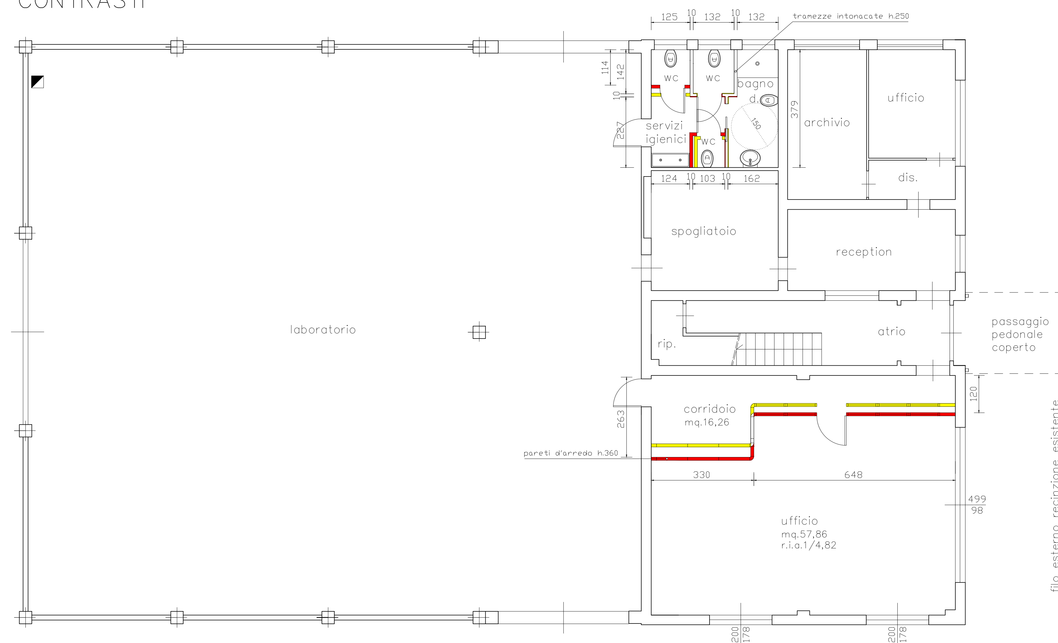
PIANO TERRA porzione oggetto d'intervento h.360
