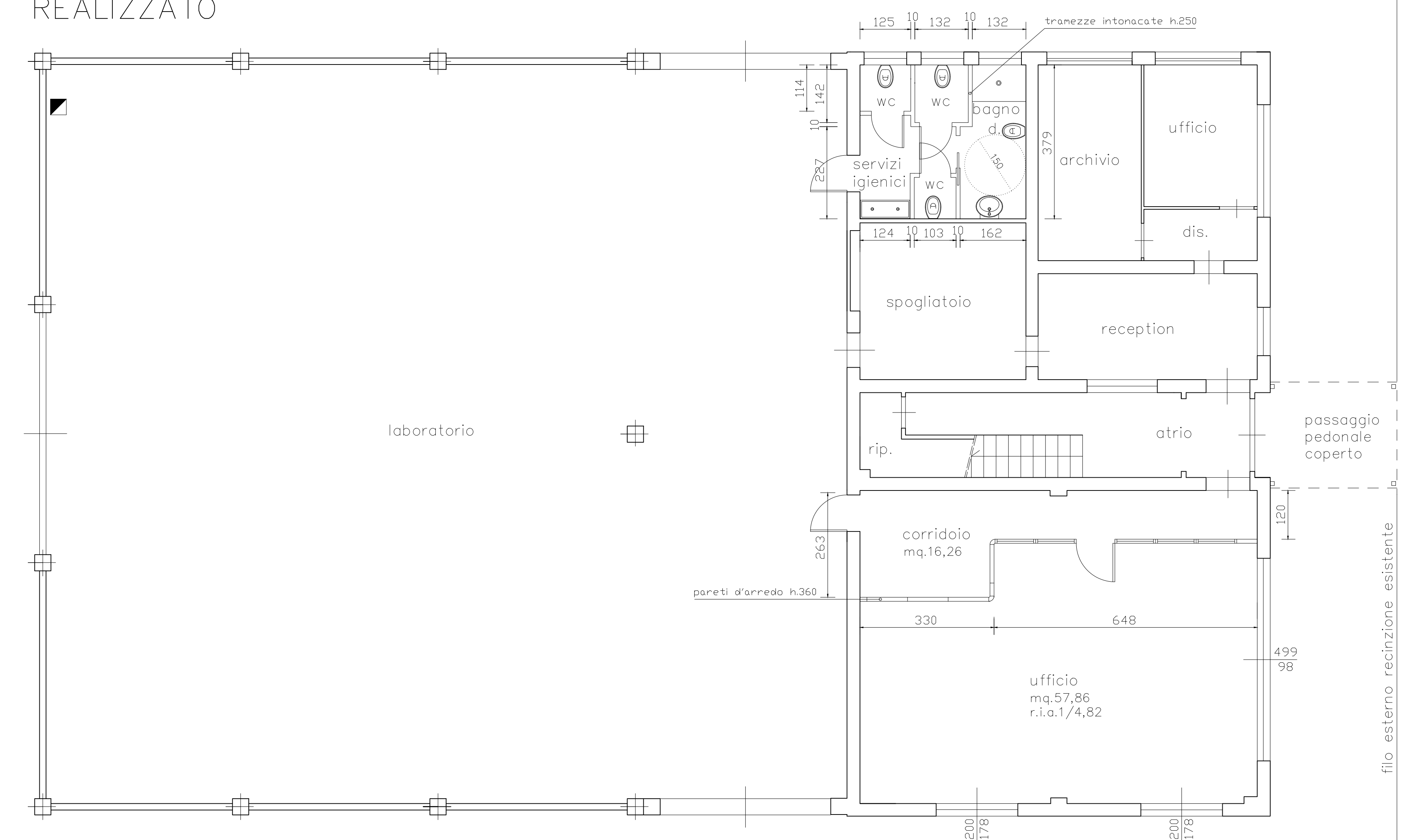
PIANO TERRA porzione oggetto d'intervento h.360
