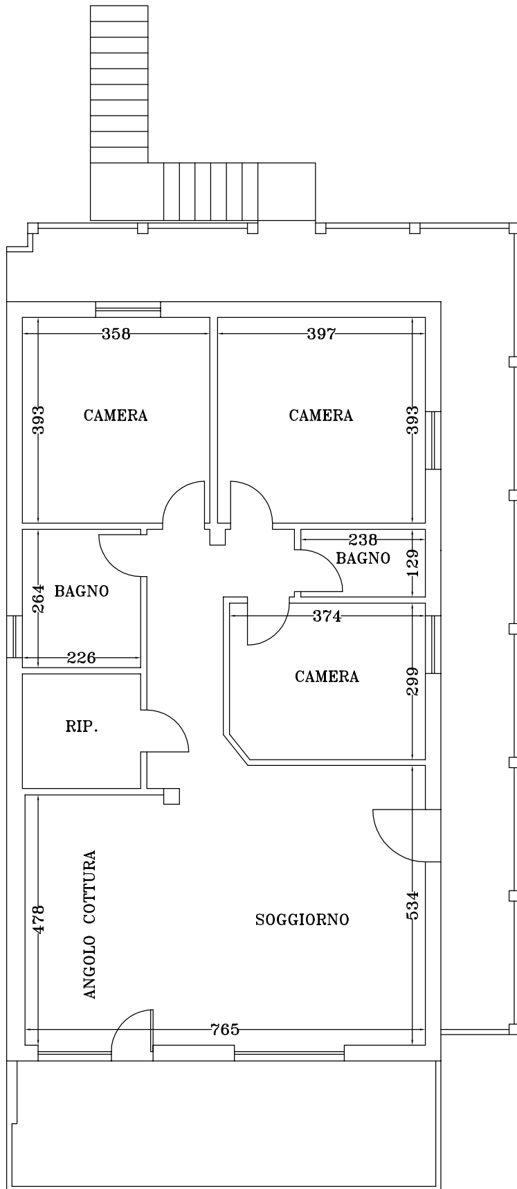
PIANO PRIMO
