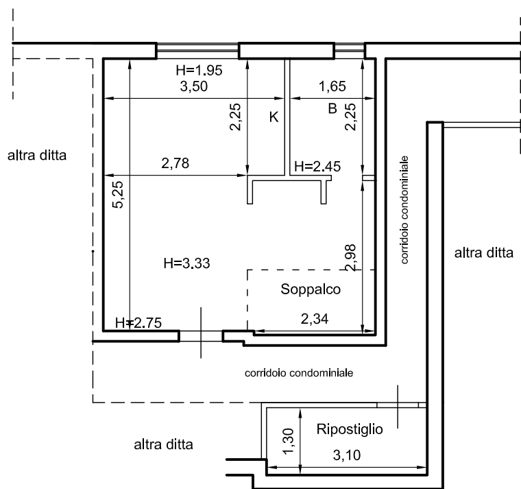
FG 5 p.IIa 158 sub 31 SCALA 1:100
