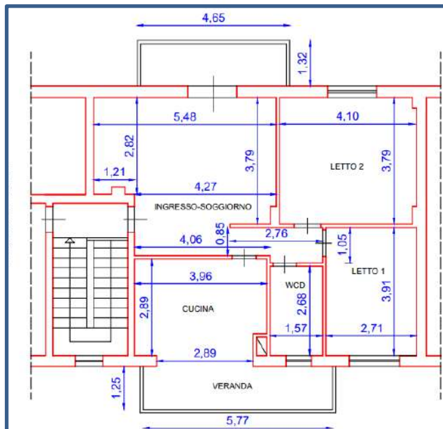
Planimetria quotata
