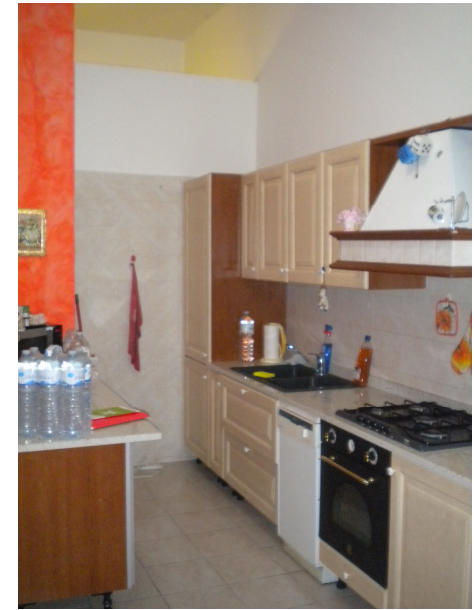
Foto 5 – Cucina
