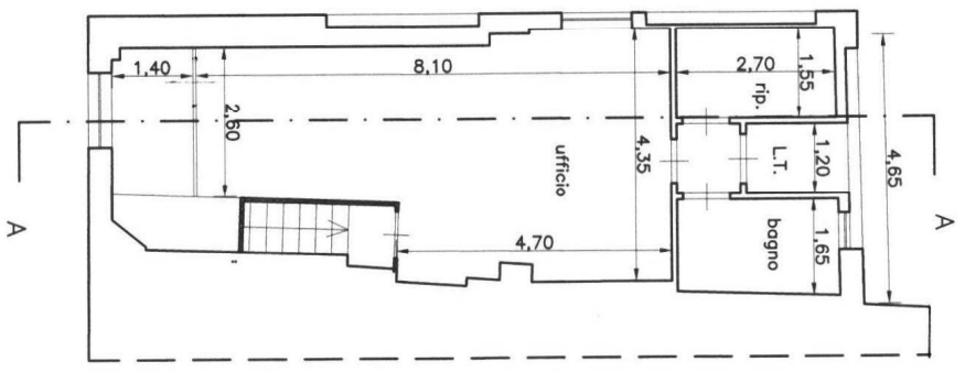
PIANO PRIMO
