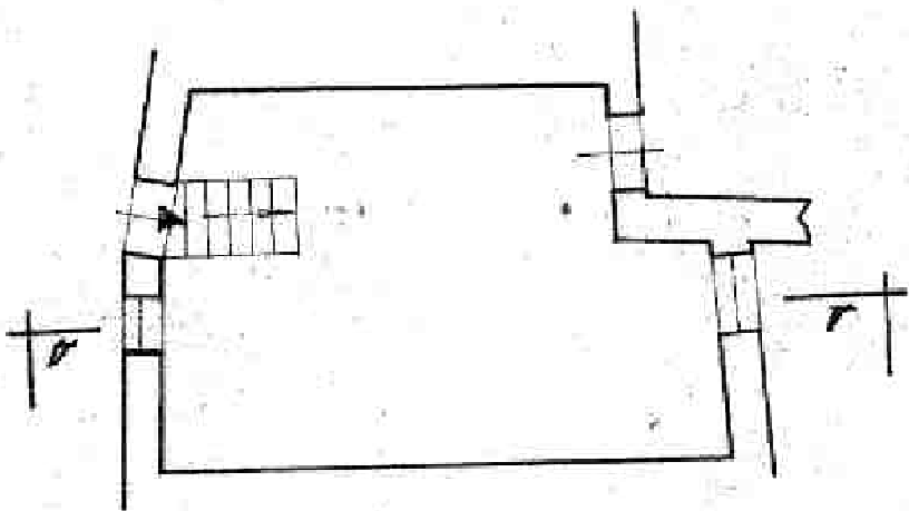
Piano Primo - stato autorizzato con L.E. n. 10 del 03/06/1968
