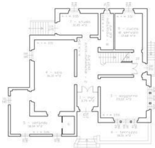
stato attuale del fabbricato 621 - piano terra
