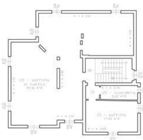
stato attuale del fabbricato 621 - piano secondo (sototetto)
