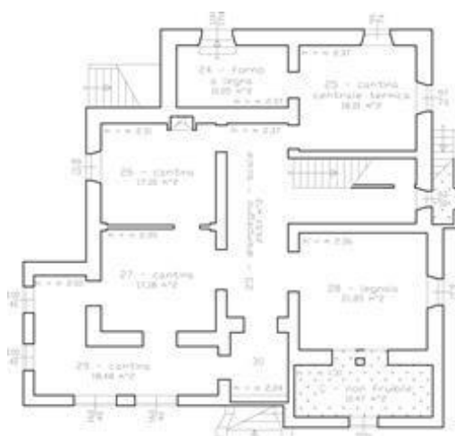
stato attuale del fabbricato 621 - piano seminterrato
