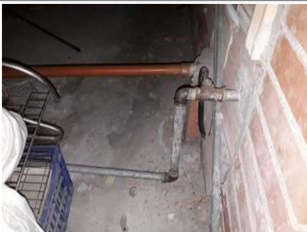
Adduzione gas sottotetto
