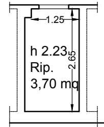
Planimetria piano 1 sottostrada stato rilevato
