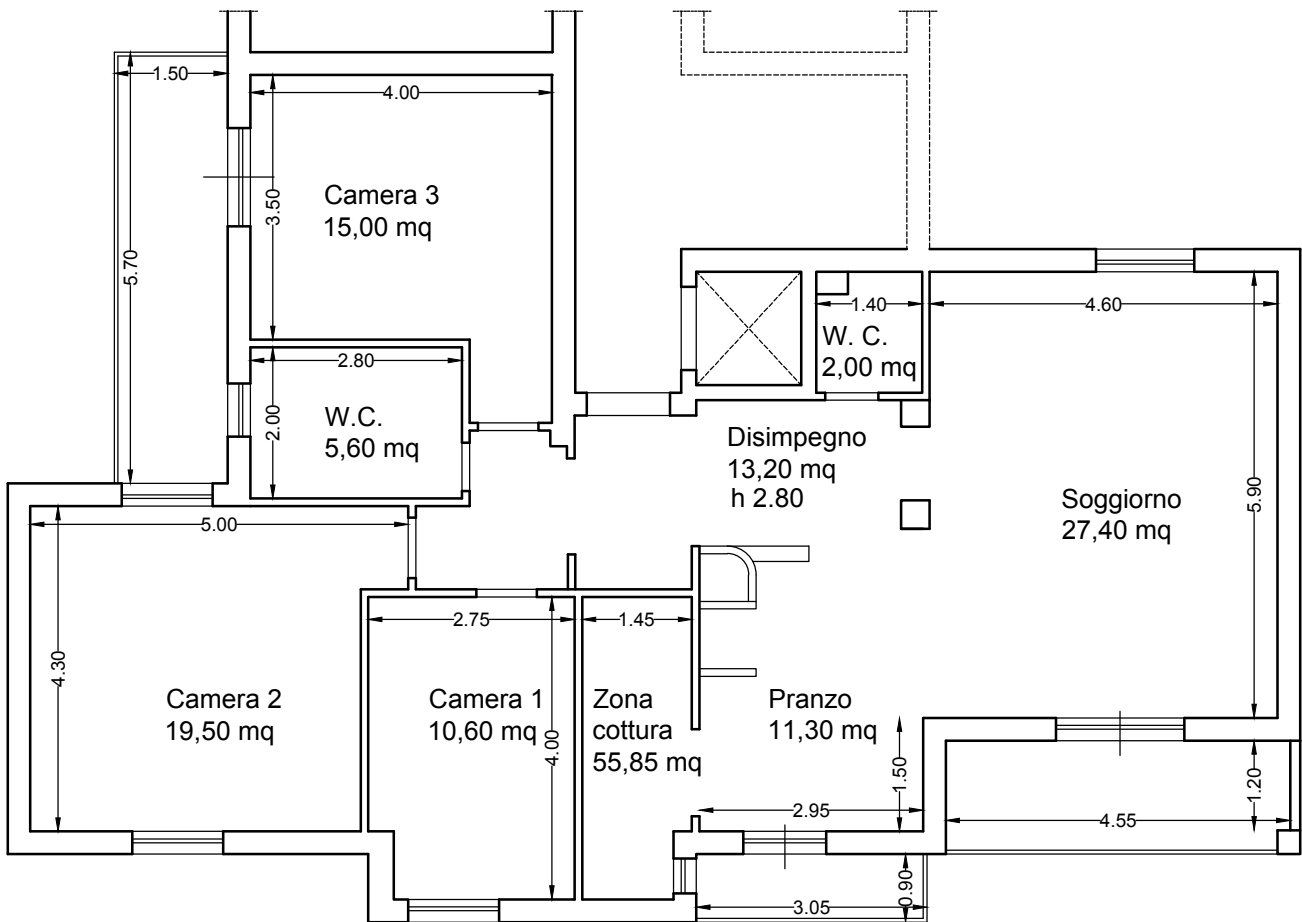
Planimetria stato rilevato
