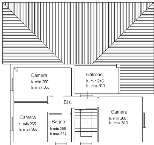
PIANO PRIMO
