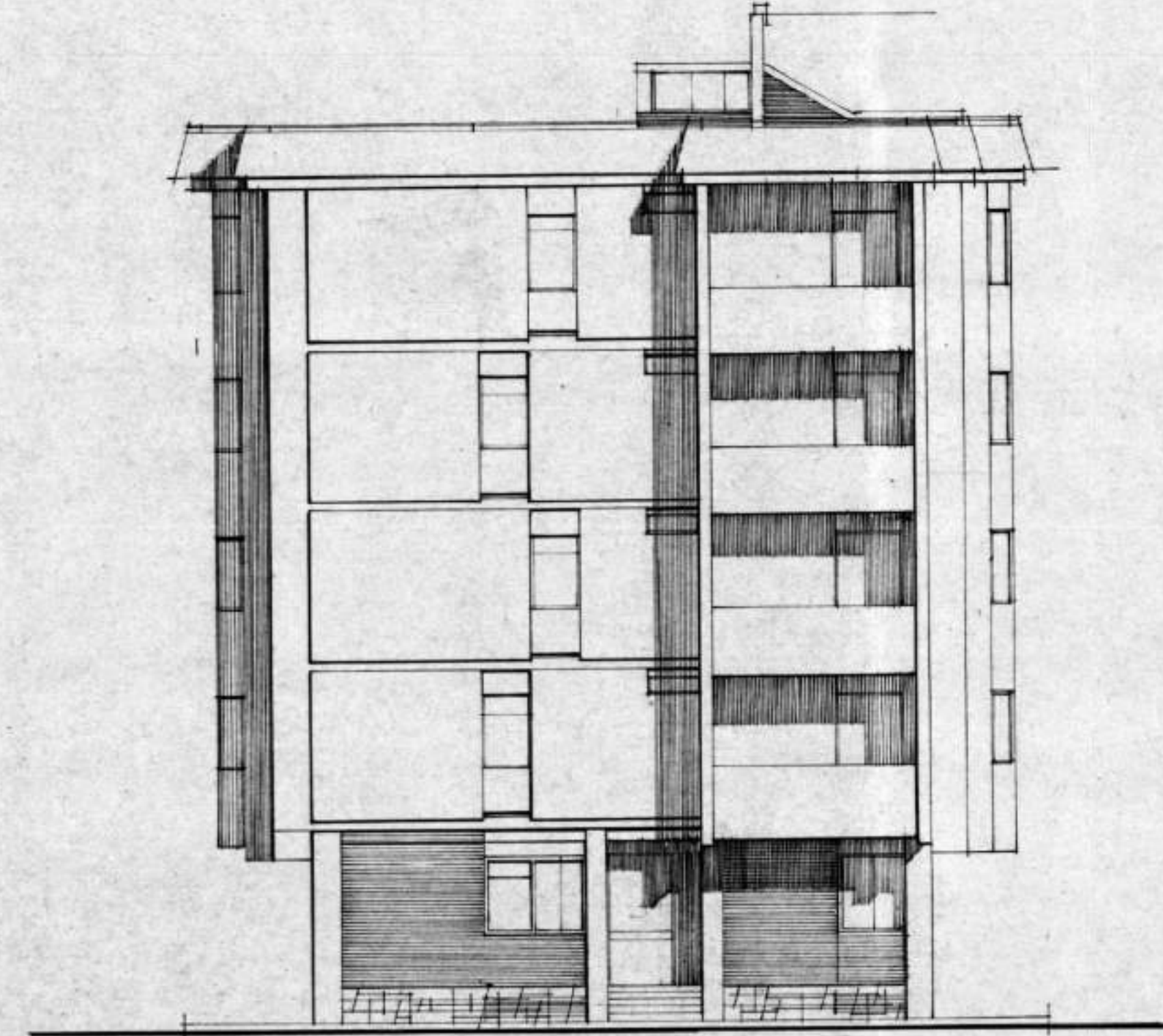
PROSPETTO SUD-EST
