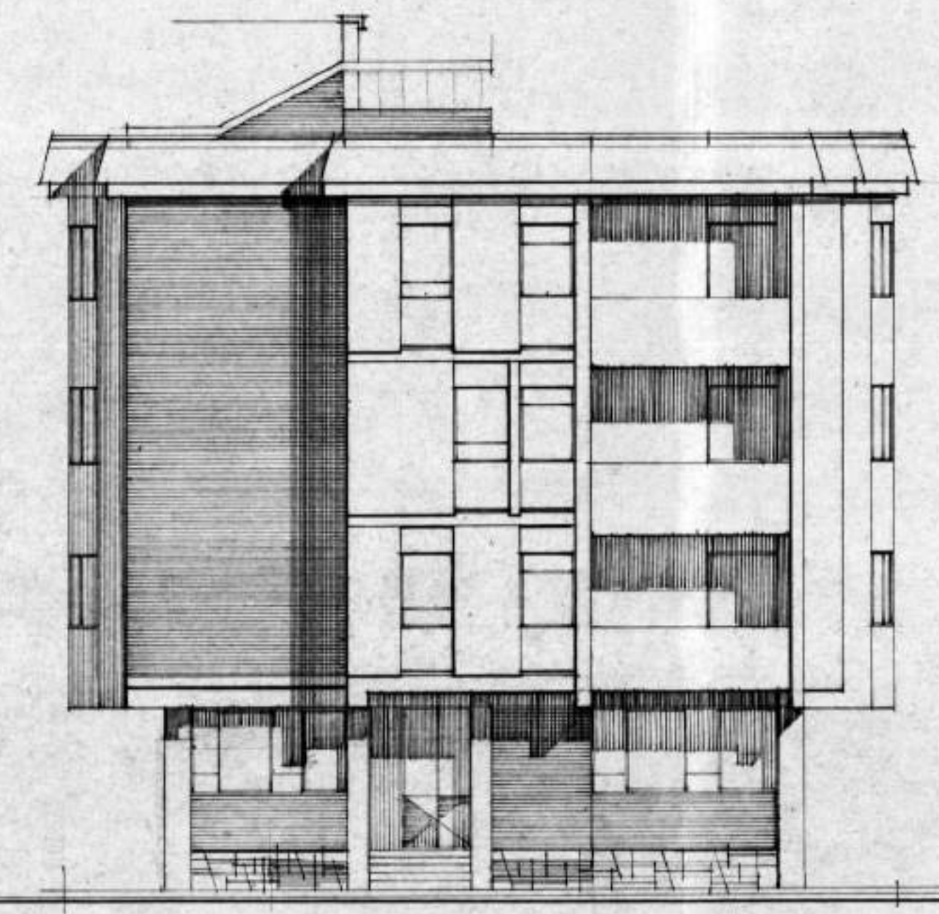
PROSPETTO NORD-EST
