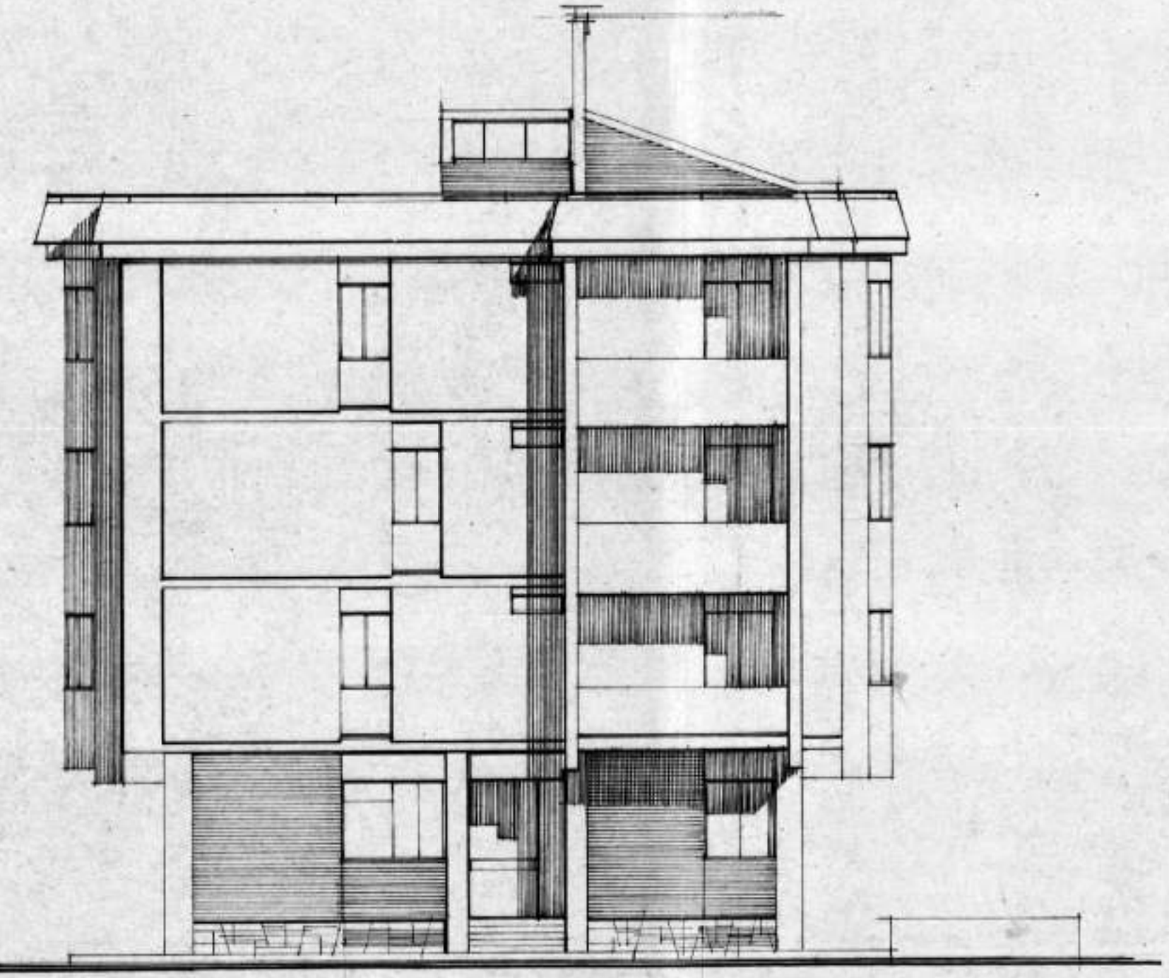
PROSPETTO SUD. EST
