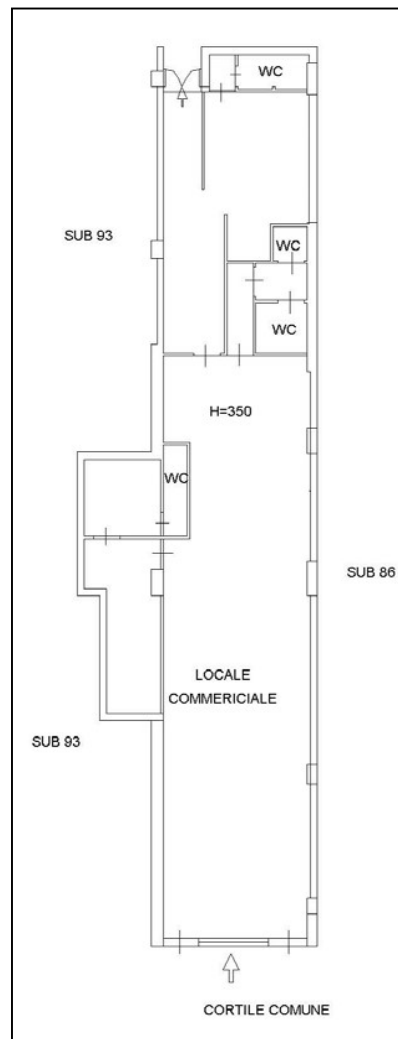
Fig. 4 – Planimetria in atti al catasto (SUB 92)
