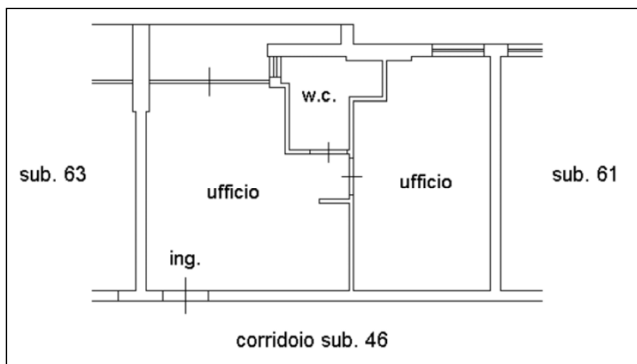
Fig. 4 – Planimetria in atti al catasto (SUB 63)
