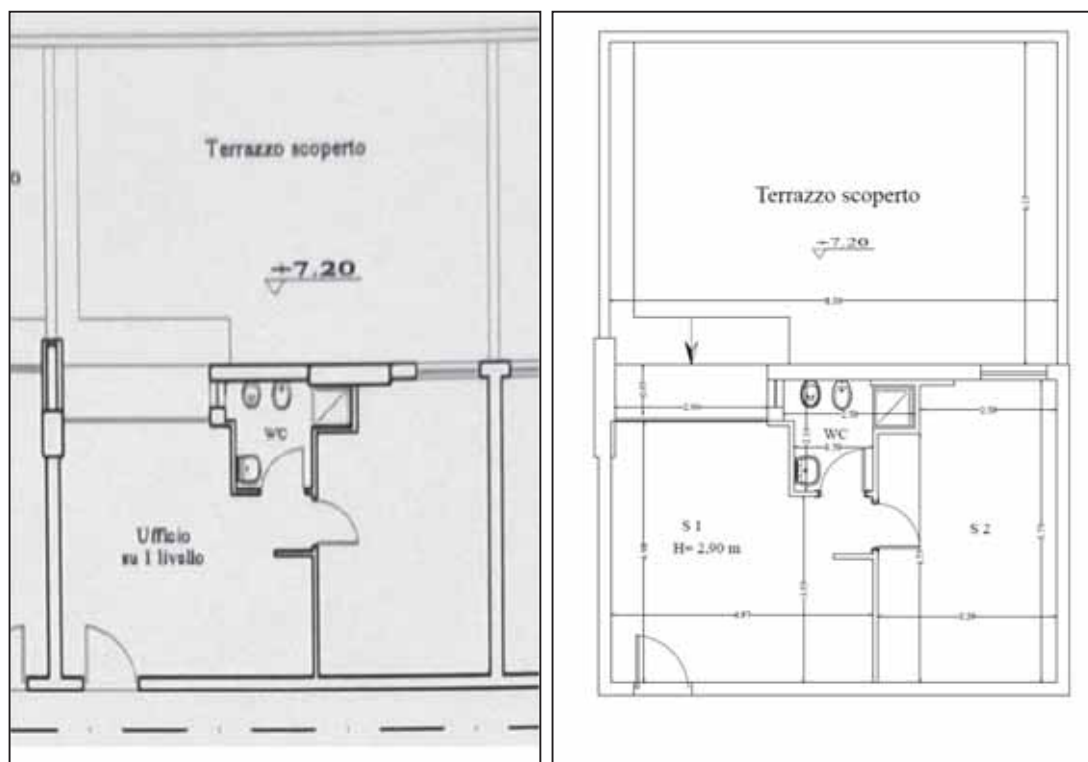
Fig. 6 - Confronto grafico PDC con lo stato dei luoghi - CONFORME
