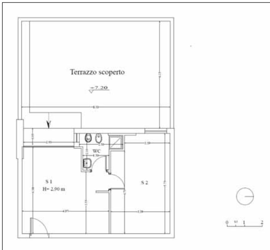
Fig. 2 - Pianta dello stato dei luoghi
