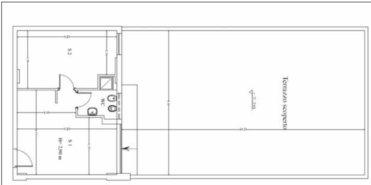
Fig. 2 - Pianta dello stato dei luoghi
