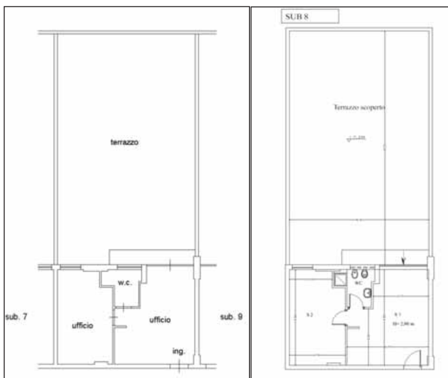
Fig. 5 – Confronto della Planimetria in atti al Catasto con lo stato dei luoghi - CONFORME
