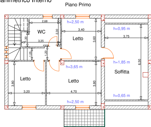
Tav. n. 5.2 Rilievo Planimetrico Interno
