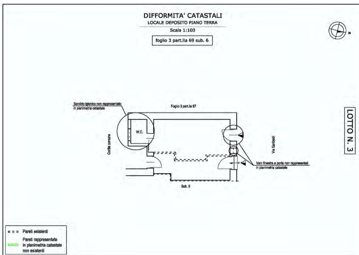
Figura 2 – Rappresentazione grafica difformità catastali unità immobiliare
