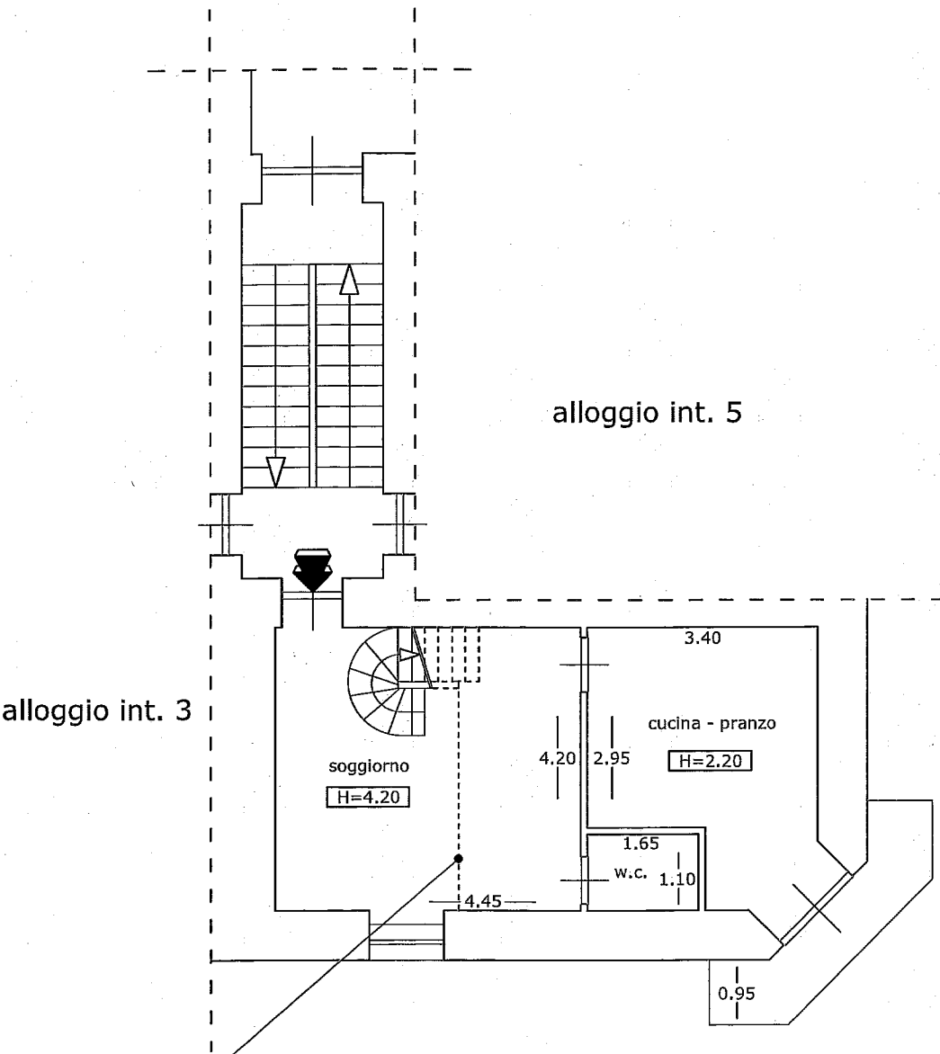
PIANTA ALLOGGIO
