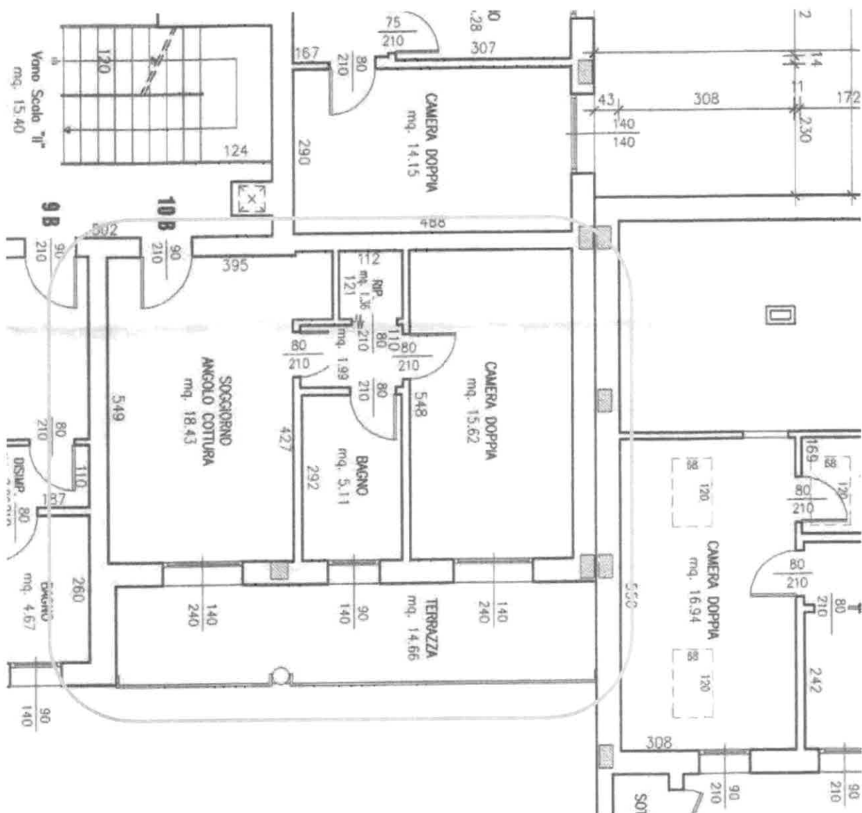
Estratto tavola 5 depositata piano terzo
