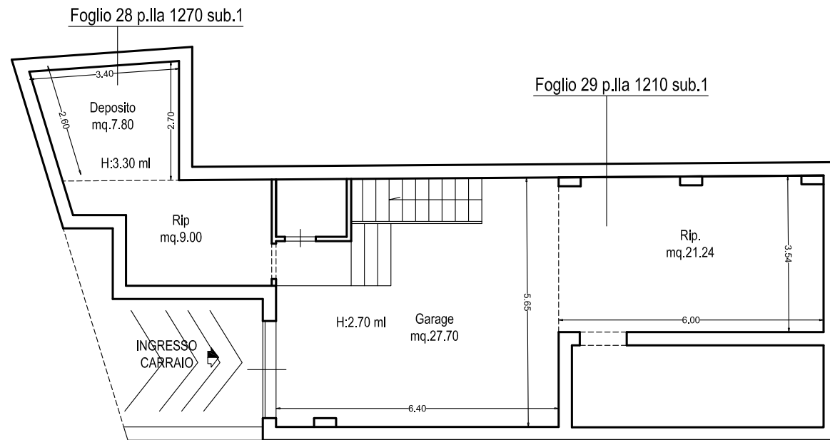
Pianta PIANO SEMINTERRATO rapp.1:100
