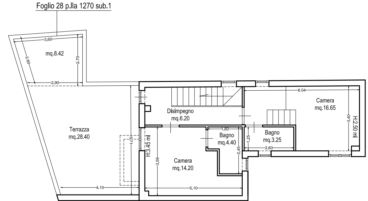
Pianta PIANO PRIMO rapp.1:100
