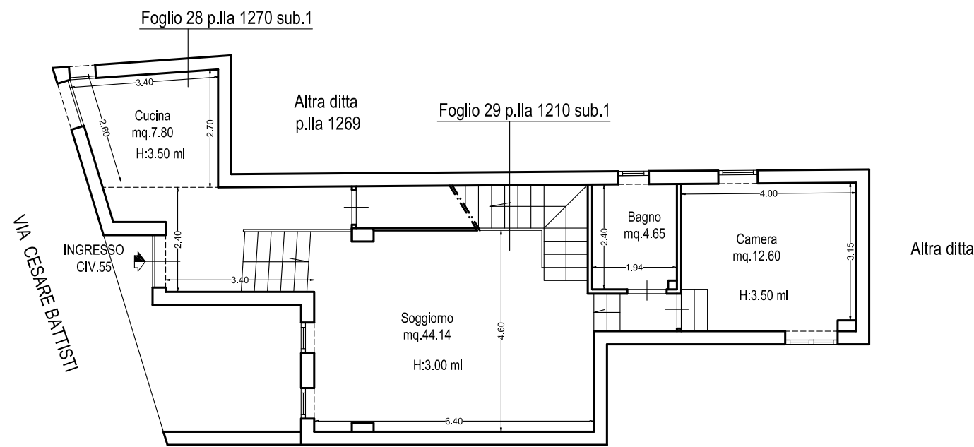
Pianta PIANO TERRA rapp.1:100
