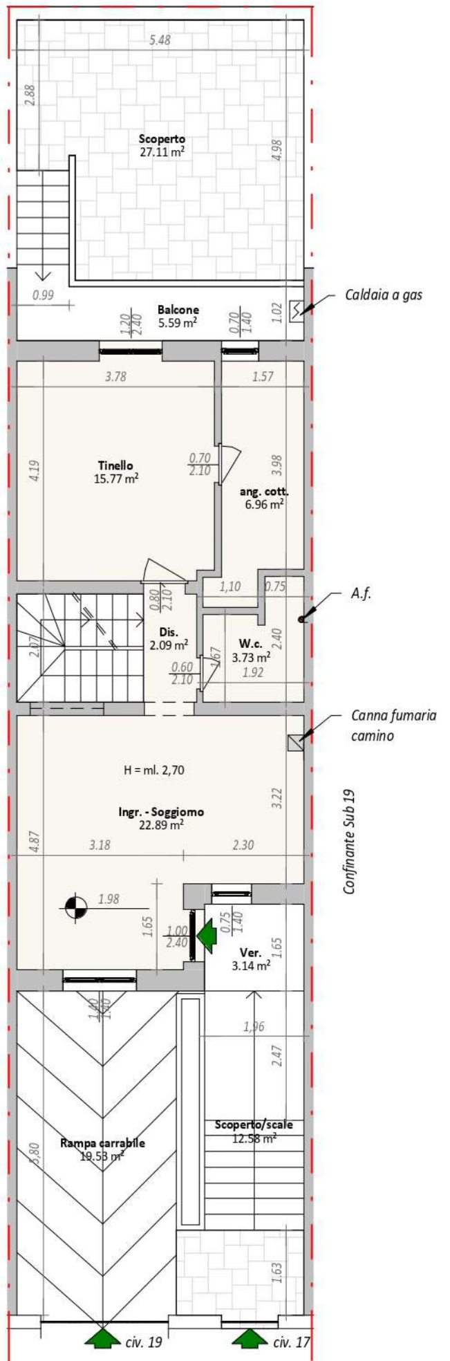
Pianta piano terra (Stato attuale) 1 : 100
