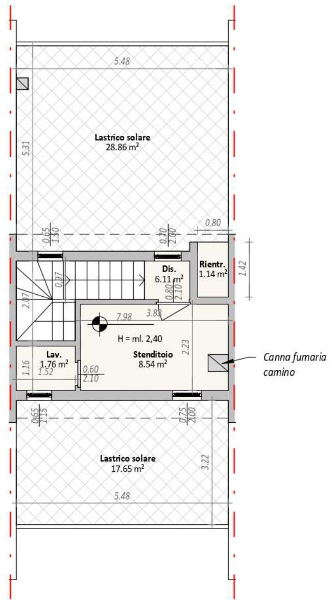
Pianta piano secondo (Stato attuale) 1 : 100
