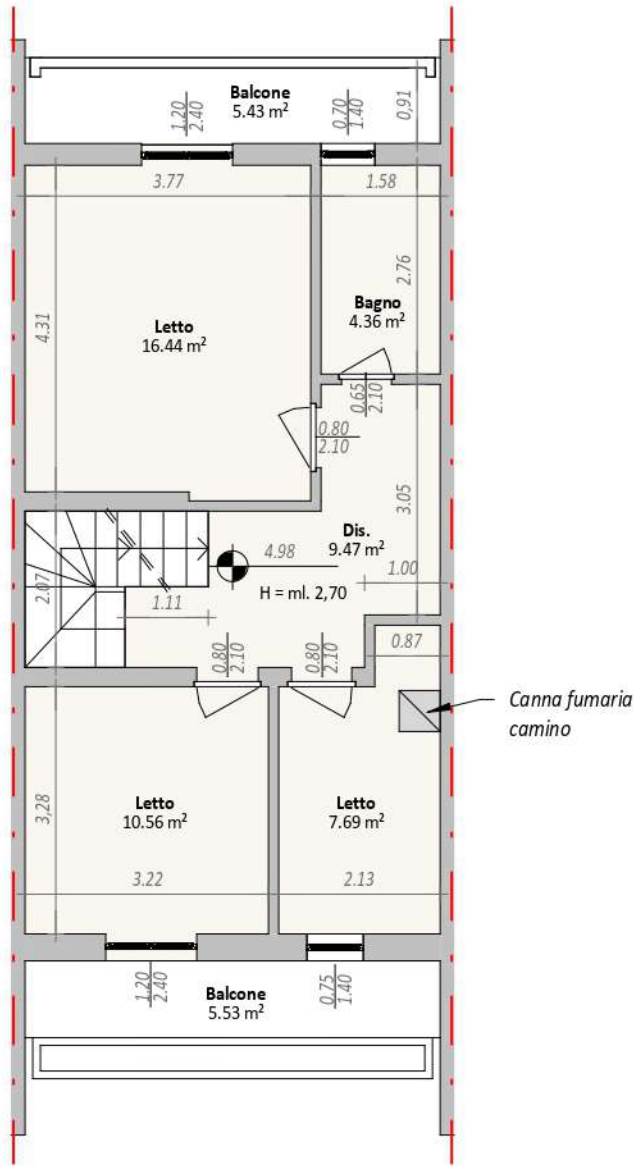
Pianta piano primo (Stato attuale) 1 : 100
