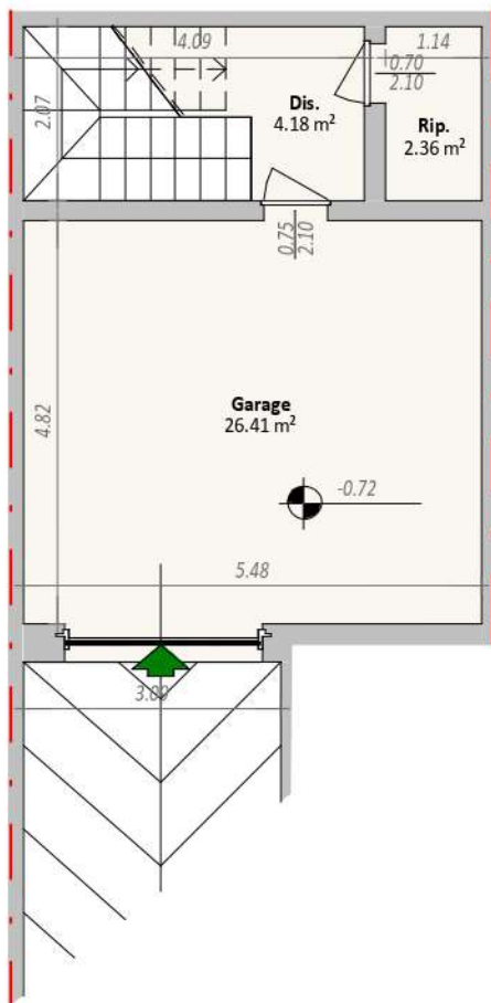
Piano piano interrato (Stato attuale) 1 : 100
